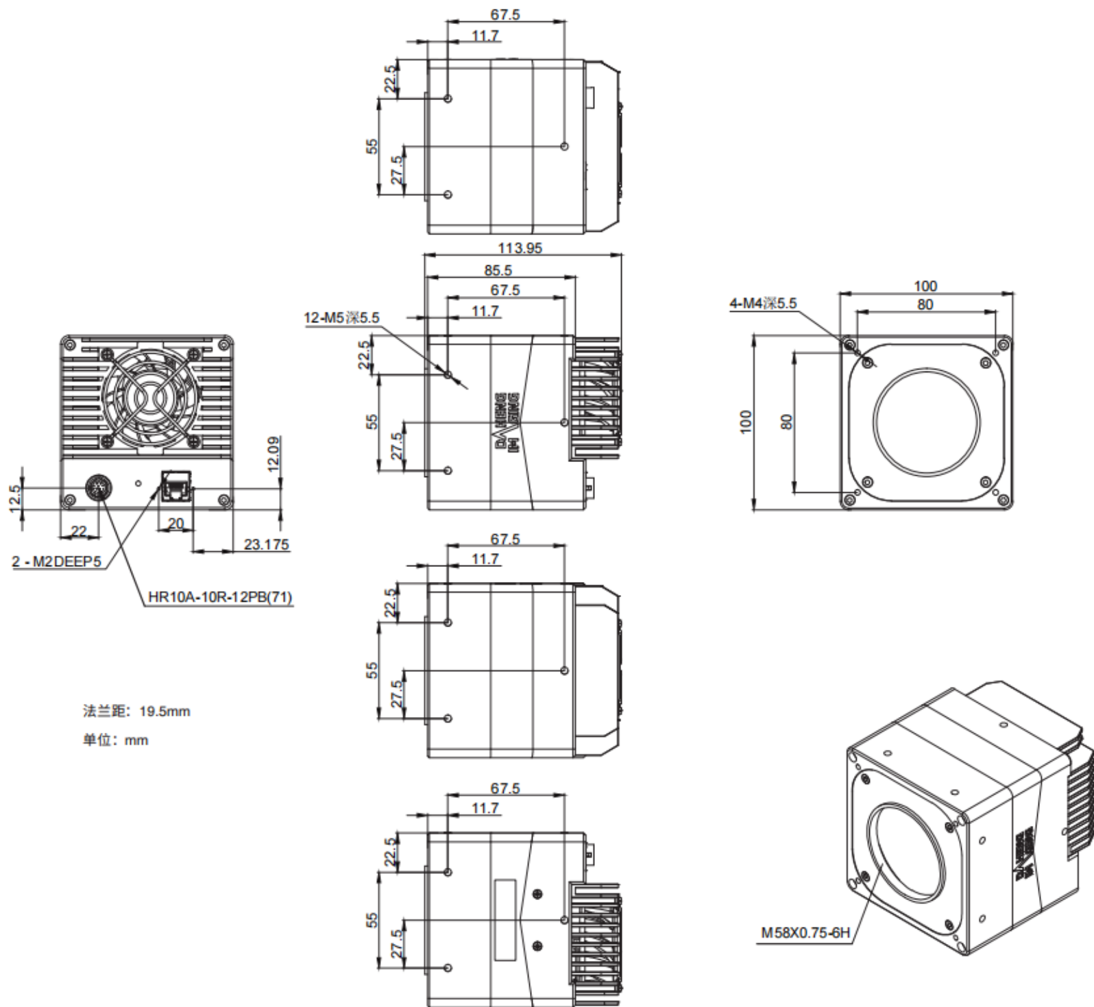
MARS-6100-18GTM/C-TF M58, M58 口 (法兰距 19.5mm)
