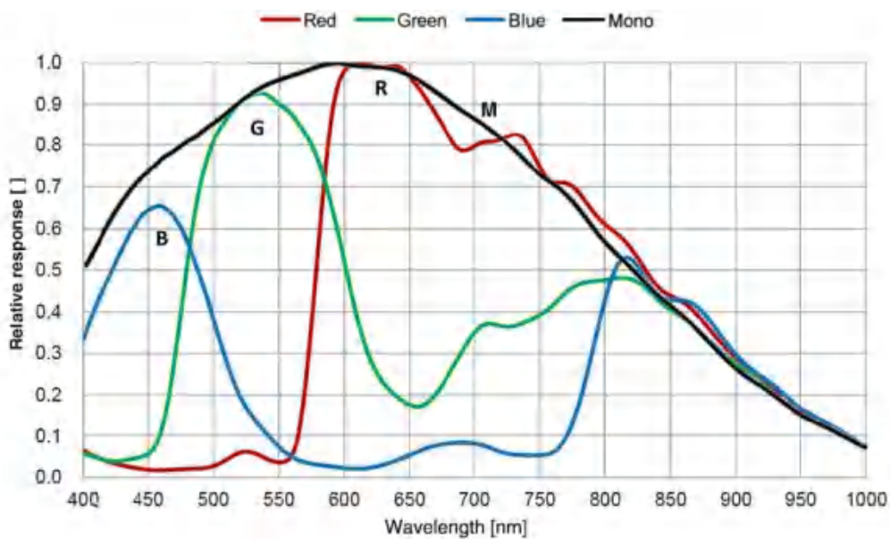
图 4-16 MER2-502-79U3M/C(-L) SENSOR 响应曲线
