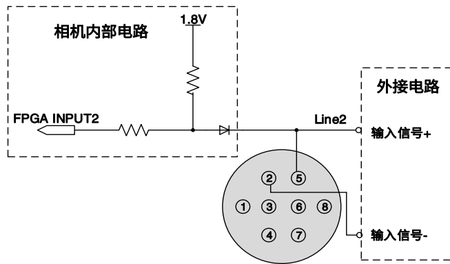
图 7-15 Line2 配置为输入引脚时相机内部等效电路 (ME2L)
