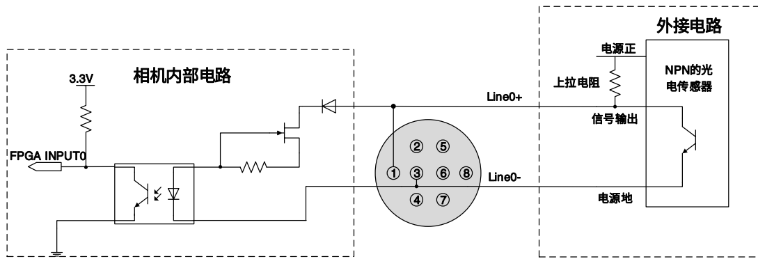
图 7-3 NPN 型光电传感器连接到光耦隔离输入电路 (MER2/ME2P/ME2L)
