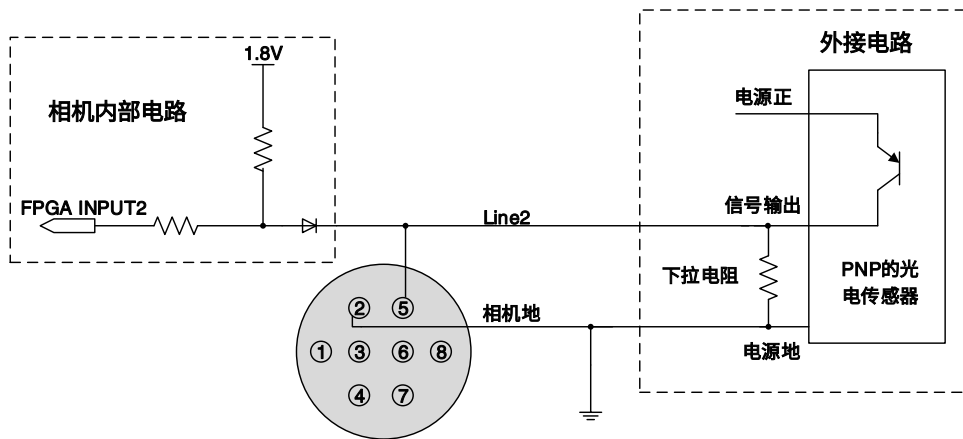
图 7-20 PNP 型光电传感器连接到 Line2 输入电路 (ME2L)
