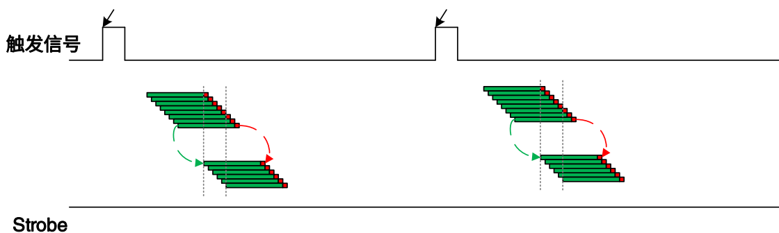
图 8-6 逐行曝光模式所有行无公共曝光时间的 Strobe 信号示意图
