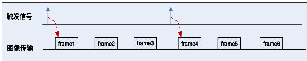
图 8-20 帧高速连拍开始触发时序图
