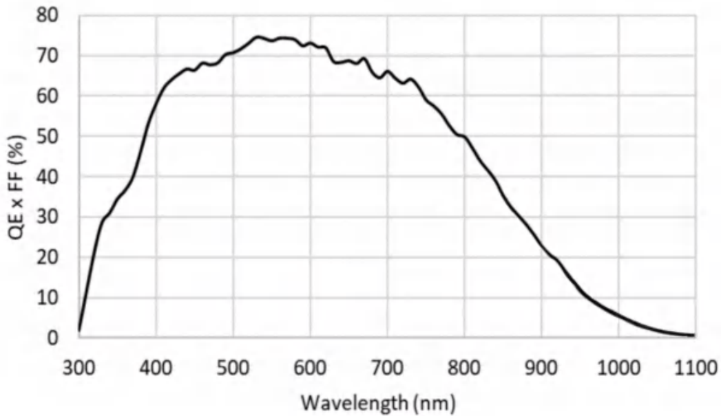
图 4-3 MER2-060-642U3M(-L) SENSOR 响应曲线
