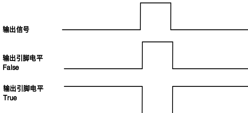
图 8-14 设置输出引脚反向
