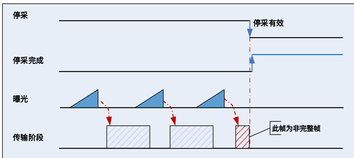
图 8-17 传输过程中停采时序图
