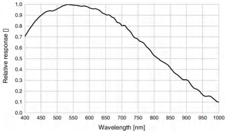
图 4-37 ME2S-2560-15U3M SENSOR 响应曲线
