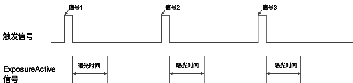
图 8-7 全局曝光模式 ExposureActive 信号示意图
