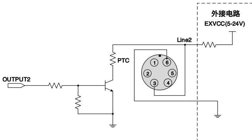
图 7-26 Line2 配置为输出引脚时相机内部等效电路 (MER2-6P/ME2S)
