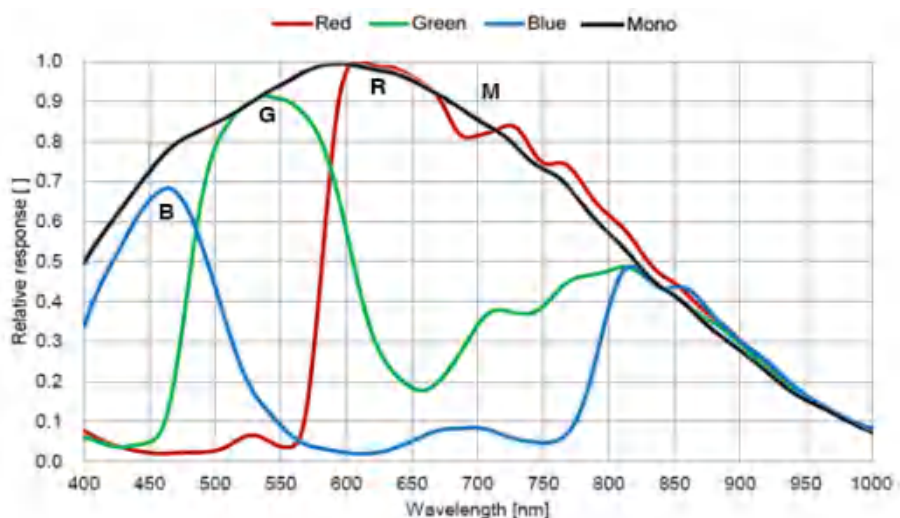
图 4-2 MER2-041-528U3M/C(-L) SENSOR 响应曲线
