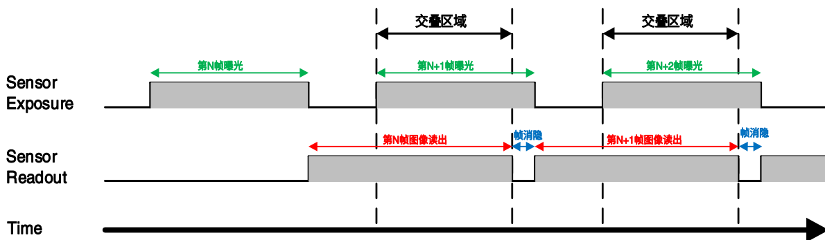
图 8-26 交叠曝光模式下曝光时序图
