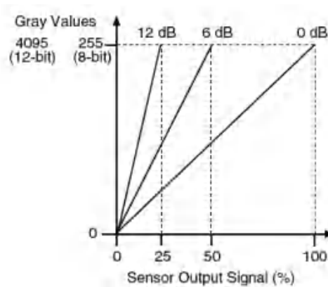
图 8-37 相机响应曲线
