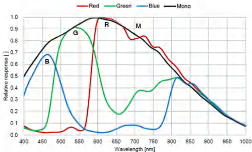
图 4-1 MER2-041-436U3M/C(-L) SENSOR 响应曲线
