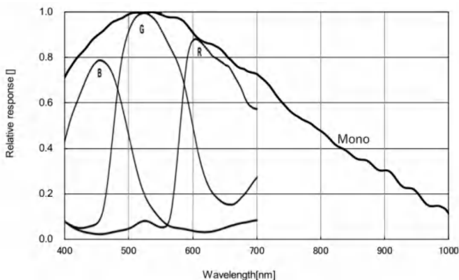
图 4-22 MER2-1220-32U3M/C(-L/-W90/-W90-S90) SENSOR 响应曲线
