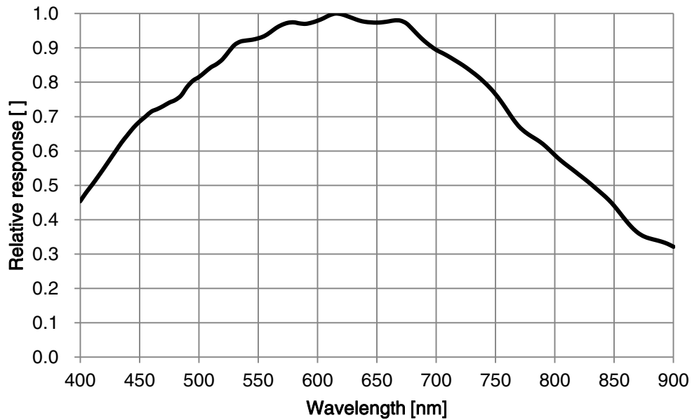
图 4-19 MER2-503-36U3M POL SENSOR 响应曲线
