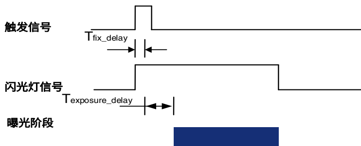
图 8-35 交叠曝光模式下曝光延迟时序图
