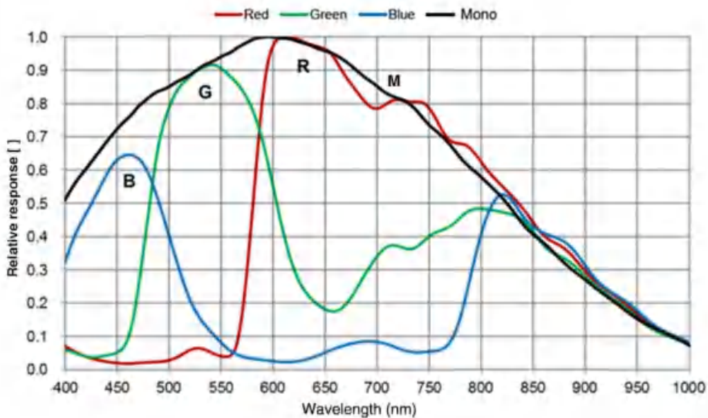
图 4-55 ME2P-1230-30U3M/C-HS SENSOR 响应曲线
