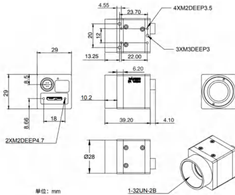
图 5-9 ME2P-U3 机械尺寸图
