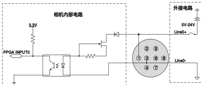
图 7-1 光耦隔离输入电路 (MER2/ME2P/ME2L)
