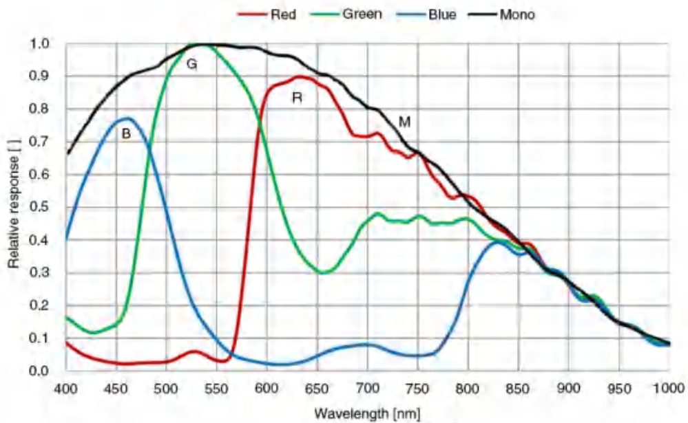
图 4-36 ME2S-2440-16U3M/C SENSOR 响应曲线
