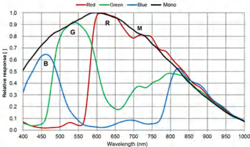
图 4-47 ME2P-1231-32U3M/C SENSOR 响应曲线
