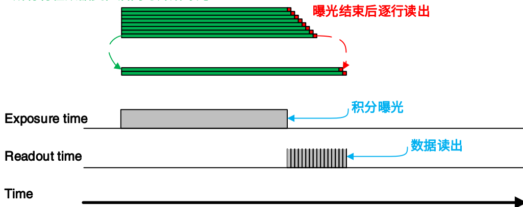
图 8-34 全局复位释放模式
