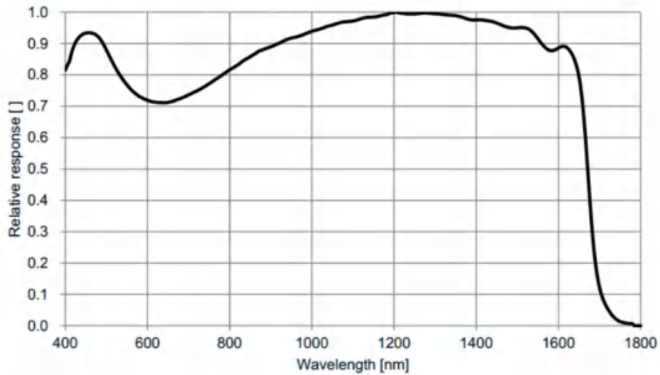
图 4-39 ME2S-138-136U3M-SWIR SENSOR 响应曲线
