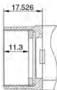
图 5-10 ME2P/MER2 C 口光学接口
