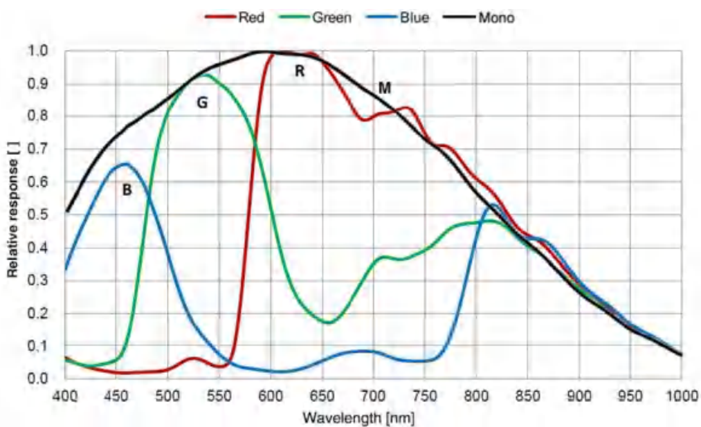
图 4-18 MER2-503-36U3M/C(-L) SENSOR 响应曲线
