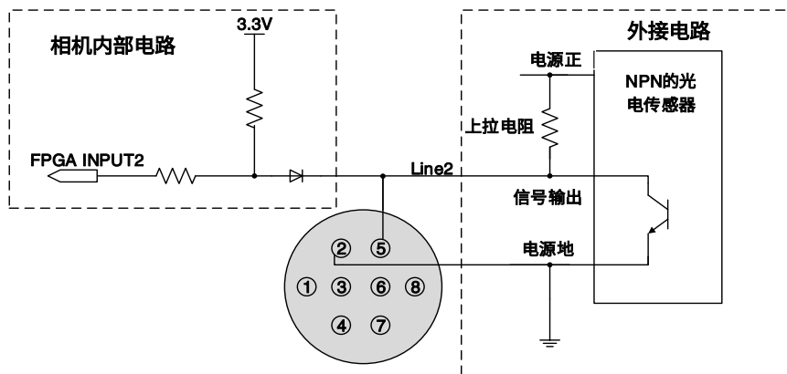
图 7-17 NPN 型光电传感器连接到 Line2 输入电路 (MER2/ME2P)
