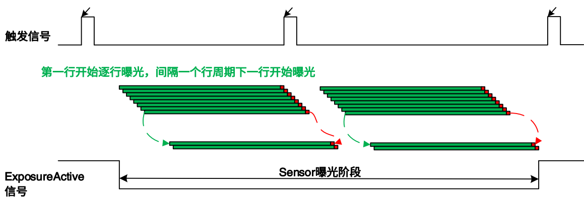
图 8-9 逐行曝光模式交叠曝光时 ExposureActive 信号示意图
