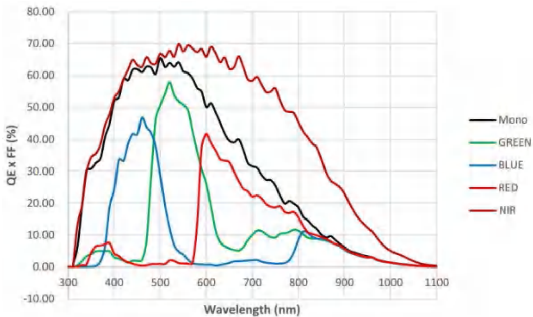
图 4-50 ME2P-2621-15U3M/C \ ME2P-2622-15U3M/C SENSOR 响应曲线
