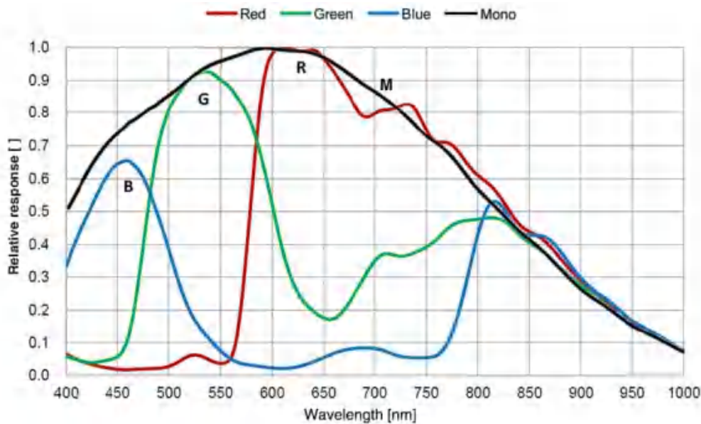
图 4-15 MER2-501-79U3M/C(-L) SENSOR 响应曲线
