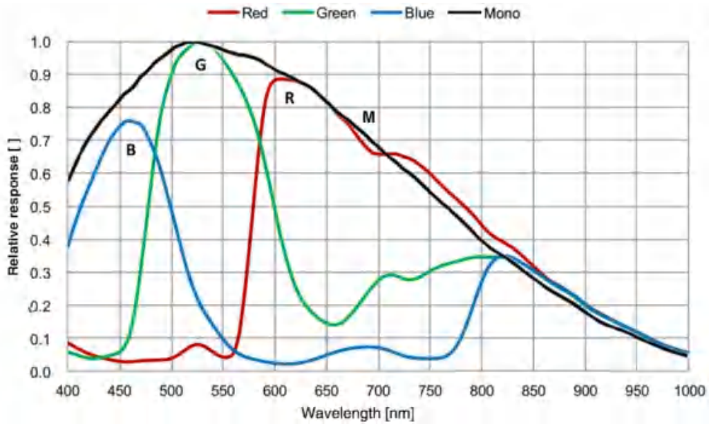
图 4-7 MER2-230-168U3M/C(-L) SENSOR 响应曲线
