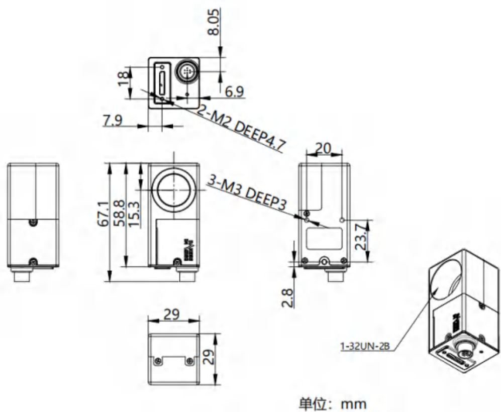
图 5-4 MER2-U3-W90-S90 机械尺寸图
