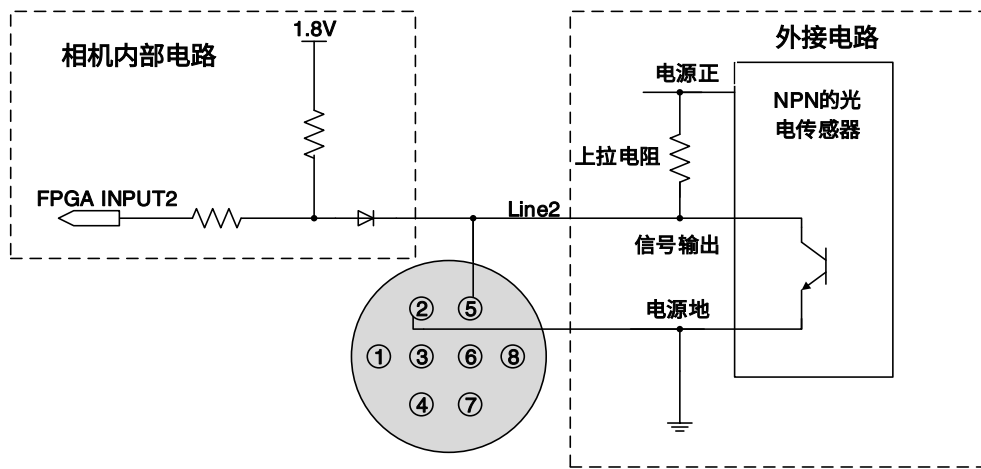
图 7-19 NPN 型光电传感器连接到 Line2 输入电路 (ME2L)
