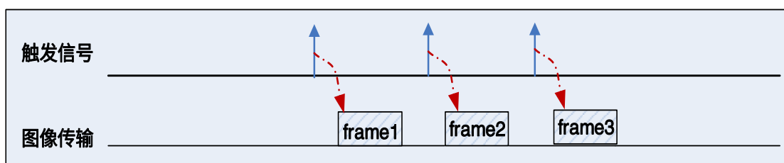
图 8-19 帧开始触发时序图
