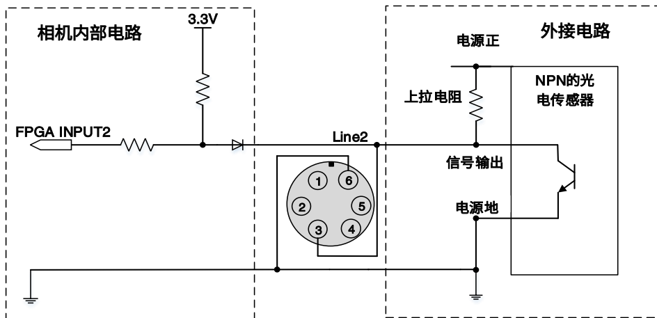
图 7-21 NPN 型光电传感器连接到 Line2 输入电路 (ME2S)
