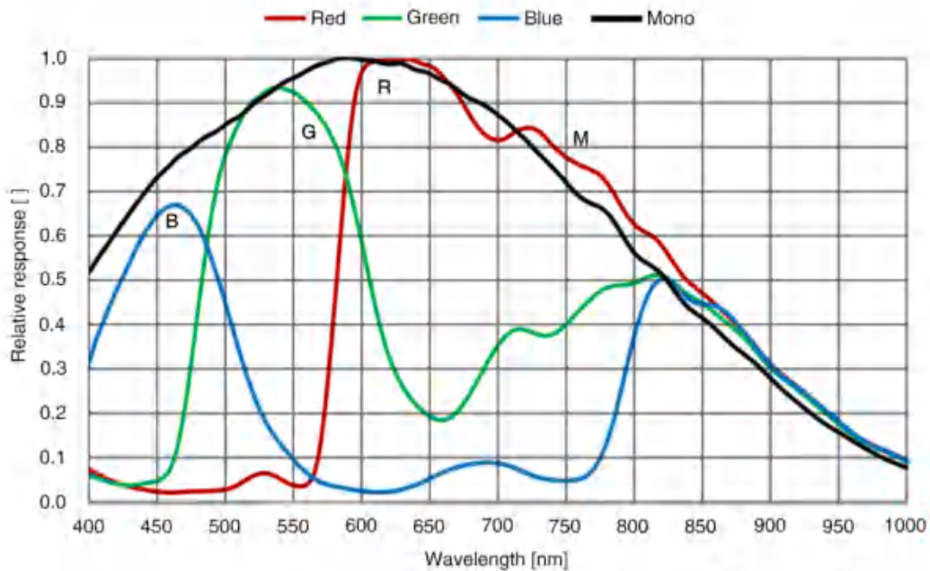
图 4-10 MER2-280-139U3M/C(-L) SENSOR 响应曲线
