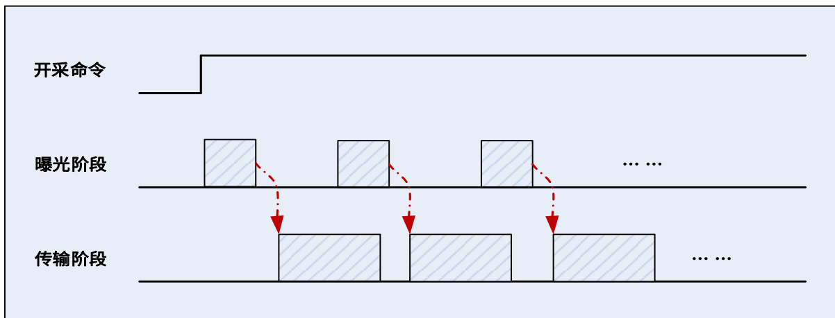
图 8-15 连续采集时序图
