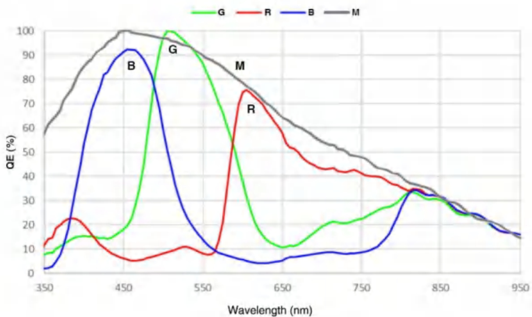
图 4-4 MER2-135-150U3M/C(-L) SENSOR 响应曲线
