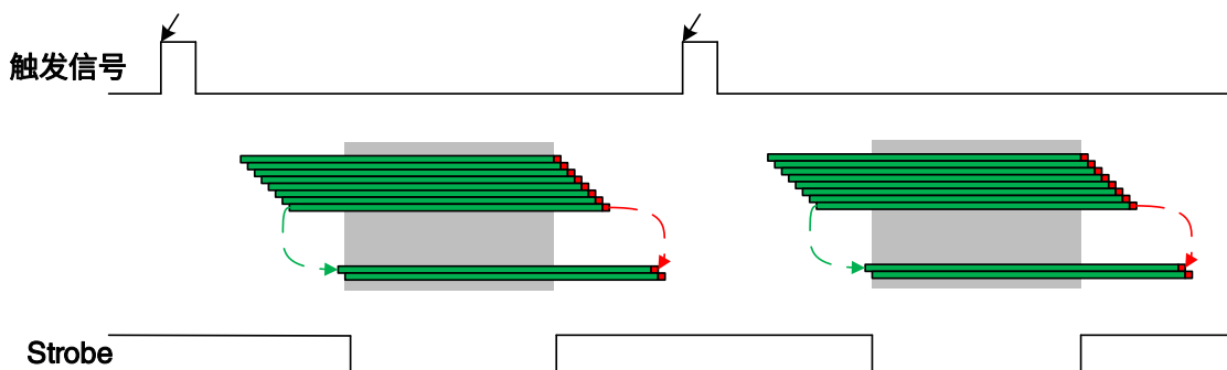
图 8-5 逐行曝光模式所有行有公共曝光时间的 Strobe 信号示意图
