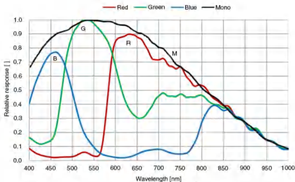
图 4-35 ME2S-2020-19U3M/C SENSOR 响应曲线
