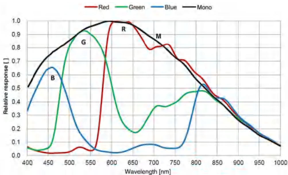
图 4-14 MER2-304-56U3M/C(-L) SENSOR 响应曲线
