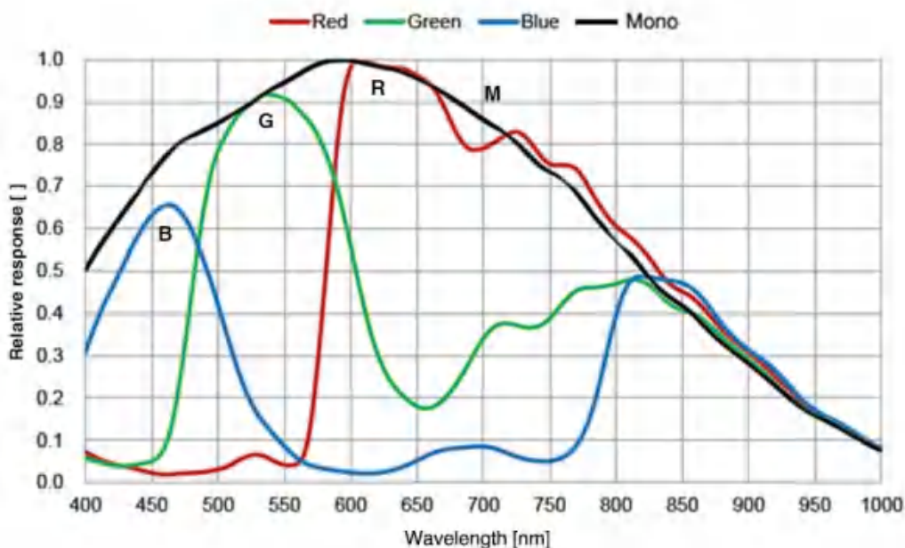
图 4-57 ME2L-161-61U3M/C(-L) SENSOR 响应曲线
