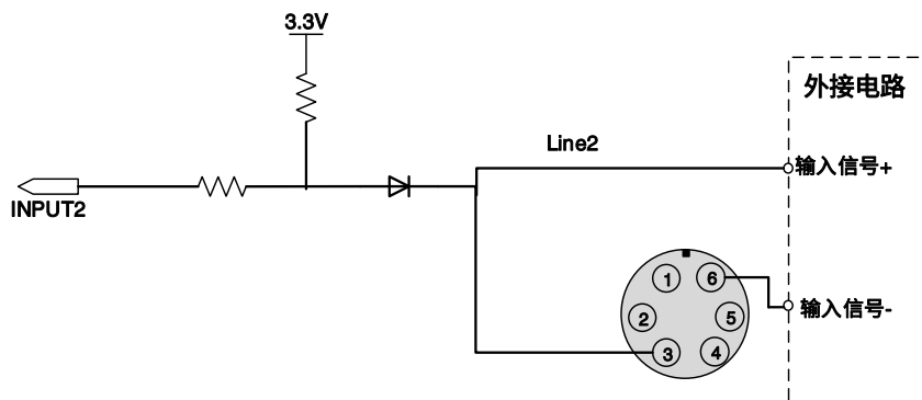
图 7-16 Line2 配置为输入引脚时相机内部等效电路 (MER2-6P/ME2S)
