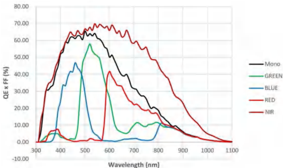
图 4-54 ME2P-2621-15U3M NIR \ ME2P-2622-15U3M NIR SENSOR 响应曲线
