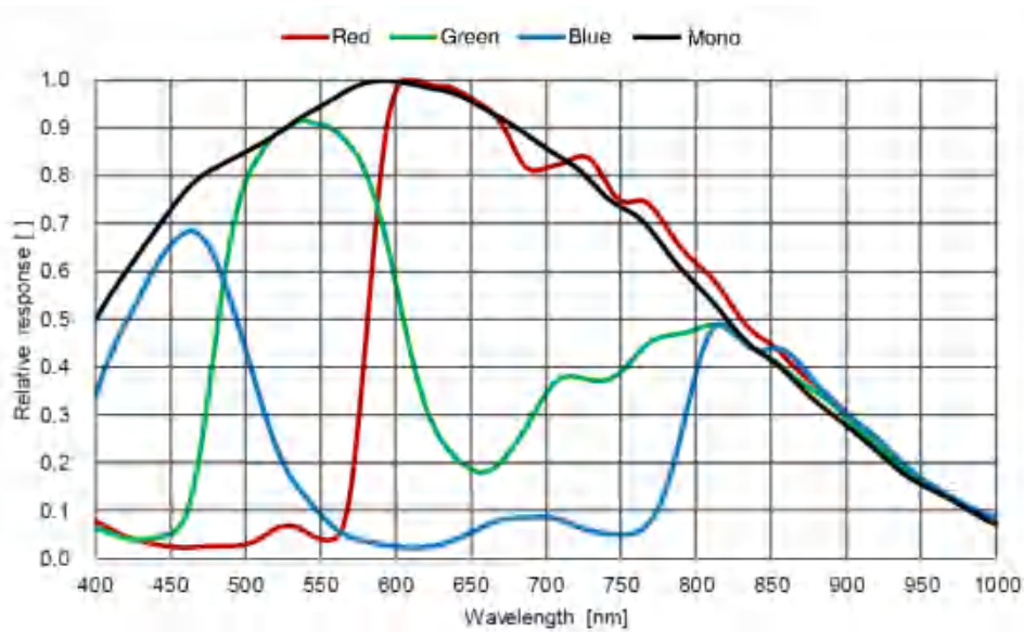
图 4-56 ME2L-042-121U3M/C(-L) SENSOR 响应曲线
