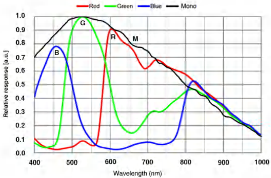
图 4-59 ME2L-830-22U3M/C(-L) SENSOR 响应曲线
