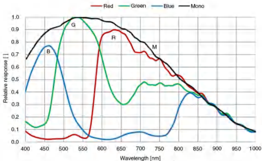
图 4-34 ME2S-1610-24U3M/C SENSOR 响应曲线
