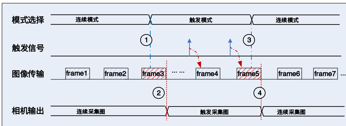
图 8-22 传输时切换触发模式
