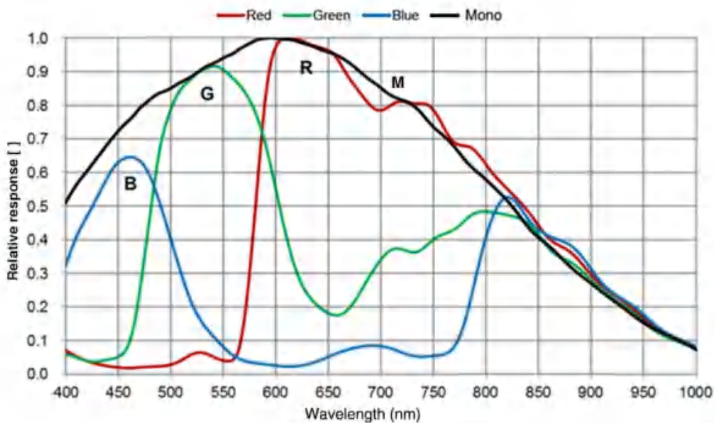
图 4-44 ME2P-883-42U3M/C SENSOR 响应曲线
