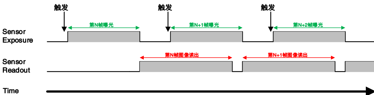
图 8-27 交叠曝光模式下触发采集曝光时序图
