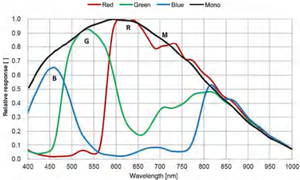
图 4-13 MER2-303-107U3M/C(-L) SENSOR 响应曲线
