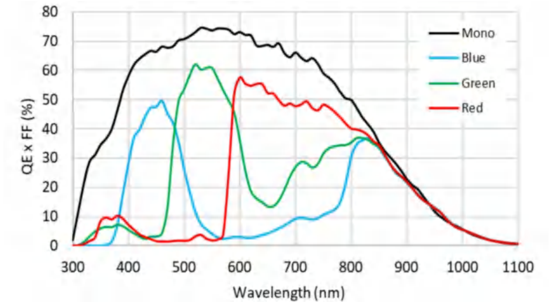
图 4-9 MER2-240-159U3M/C(-L) SENSOR 响应曲线
