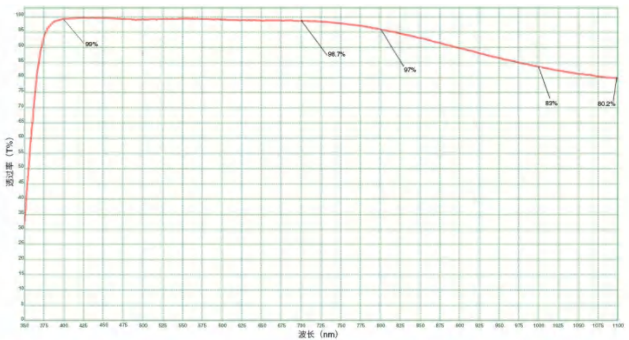
图 6-2 水星二代黑白相机滤色片透过率曲线
