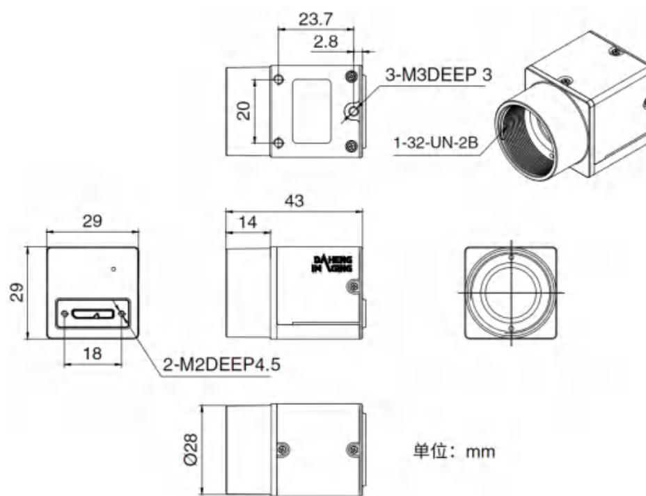
图 5-2 MER2-U3-L 机械尺寸图
