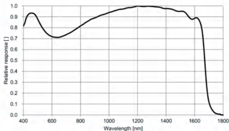
图 4-38 ME2S-033-262U3M-SWIR SENSOR 响应曲线
