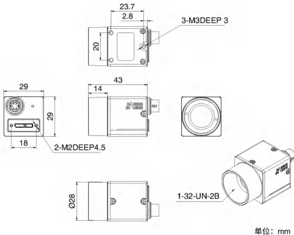
图 5-5 MER2-U3-6P 机械尺寸图
