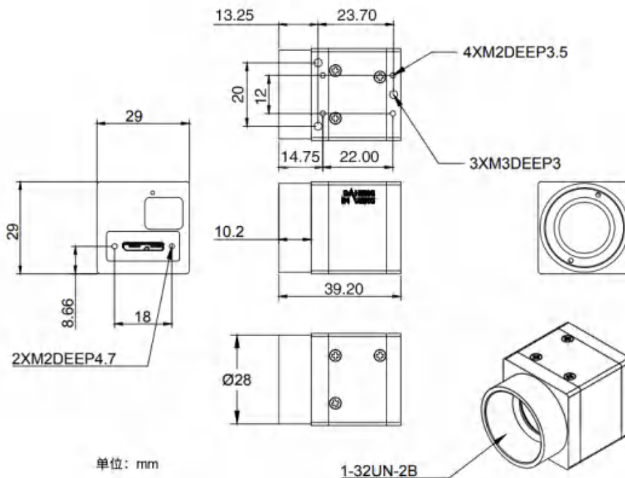
图 5-115-9 ME2L-U3-L 机械尺寸图
