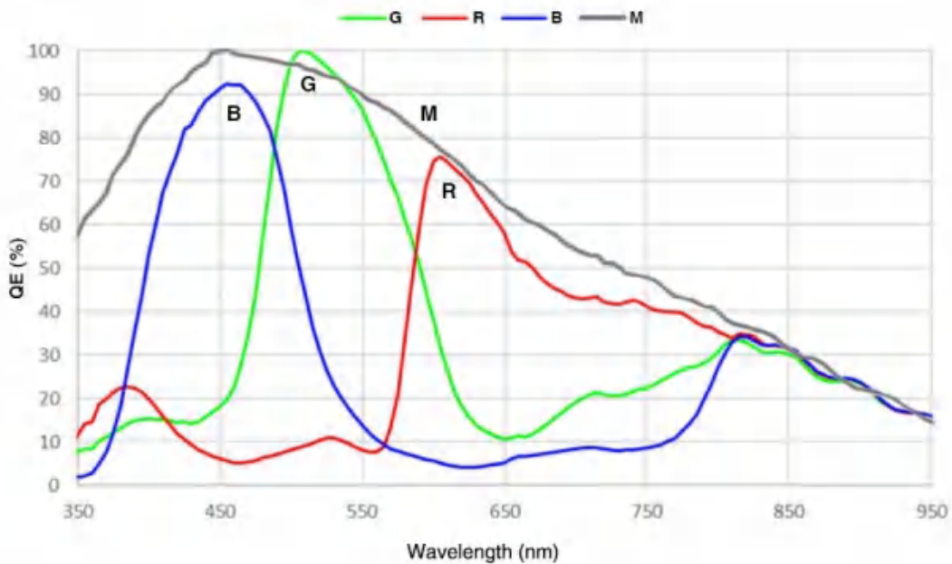
图 4-5 MER2-135-208U3M/C(-L) SENSOR 响应曲线
