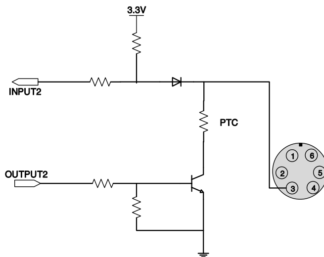
图 7-13 Line2 (双向) 电路 (MER2-6P/ME2S)
