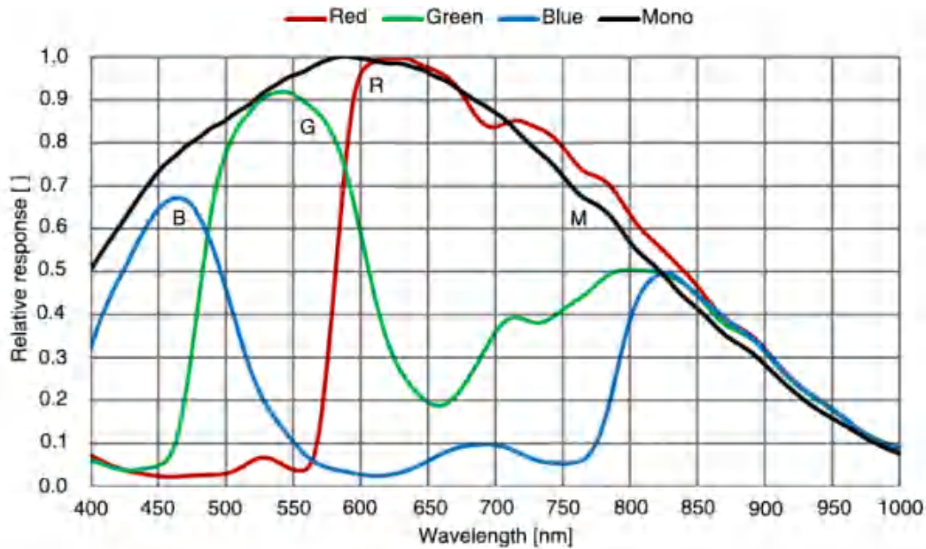
图 4-41 ME2P-170-210U3M/C SENSOR 响应曲线
