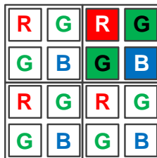
图 8-50 彩色相机水平垂直 Binning 系数 2x2
