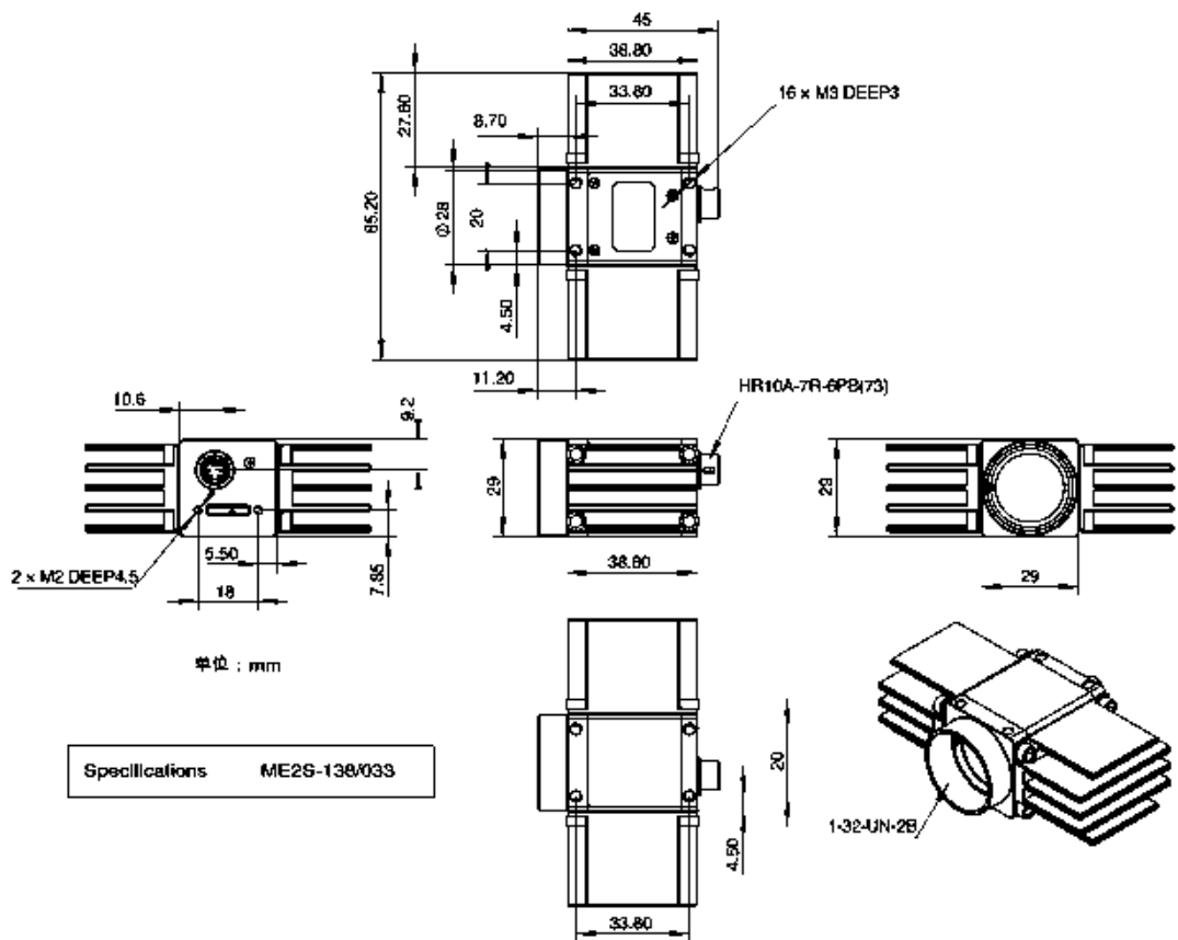
图 5-8 ME2S-U3 机械尺寸图 (含散热翅)
