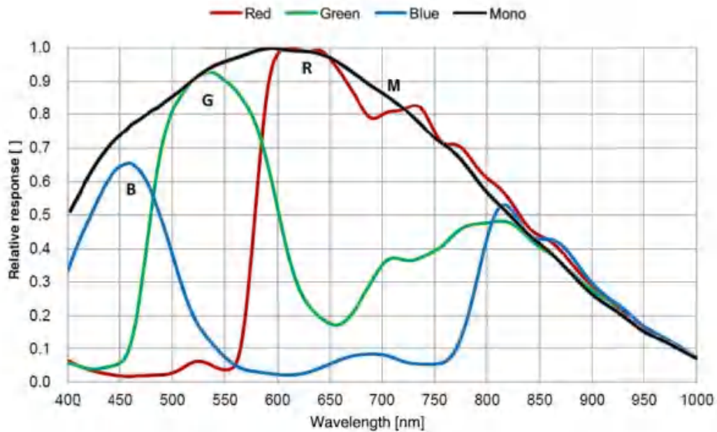
图 4-11 MER2-301-125U3M/C(-L) SENSOR 响应曲线
