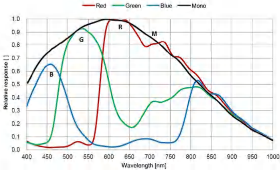
图 4-27 MER2-301-125U3M/C(-L)-HS SENSOR 响应曲线
