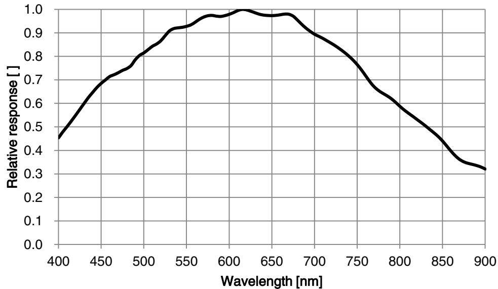
图 4-17 MER2-502-79U3M POL SENSOR 响应曲线
