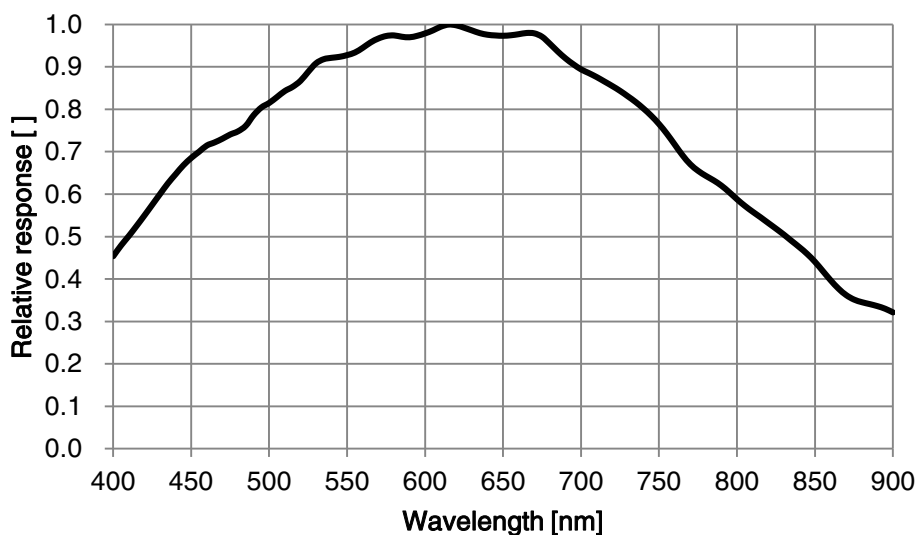
图 4-29 MER2-502-79U3M-HS POL SENSOR 响应曲线
