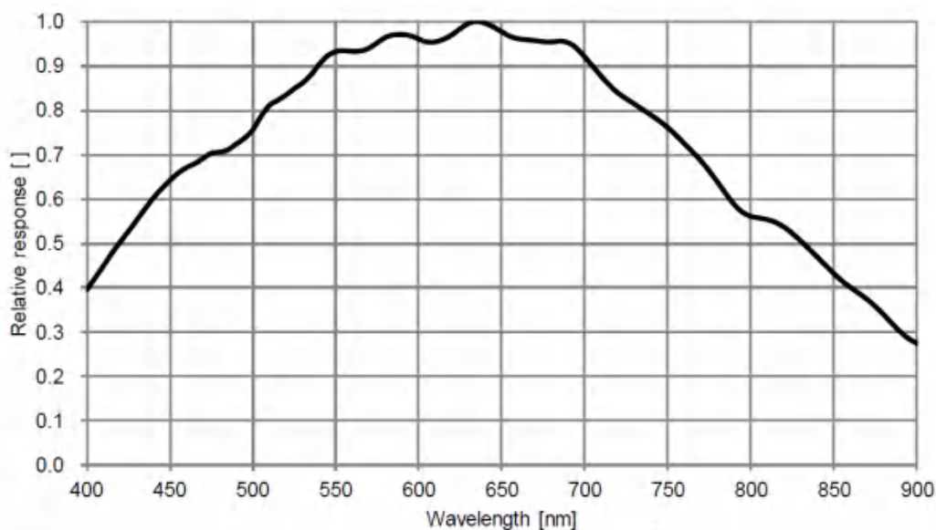
图 4-48 ME2P-1231-32U3M POL SENSOR 响应曲线
