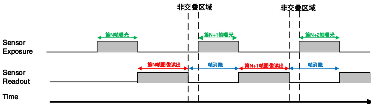
图 8-24 非交叠曝光模式下曝光时序图
