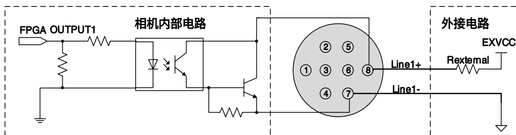
图 7-8 光耦隔离输出电路 (MER2/ME2P/ME2L)
