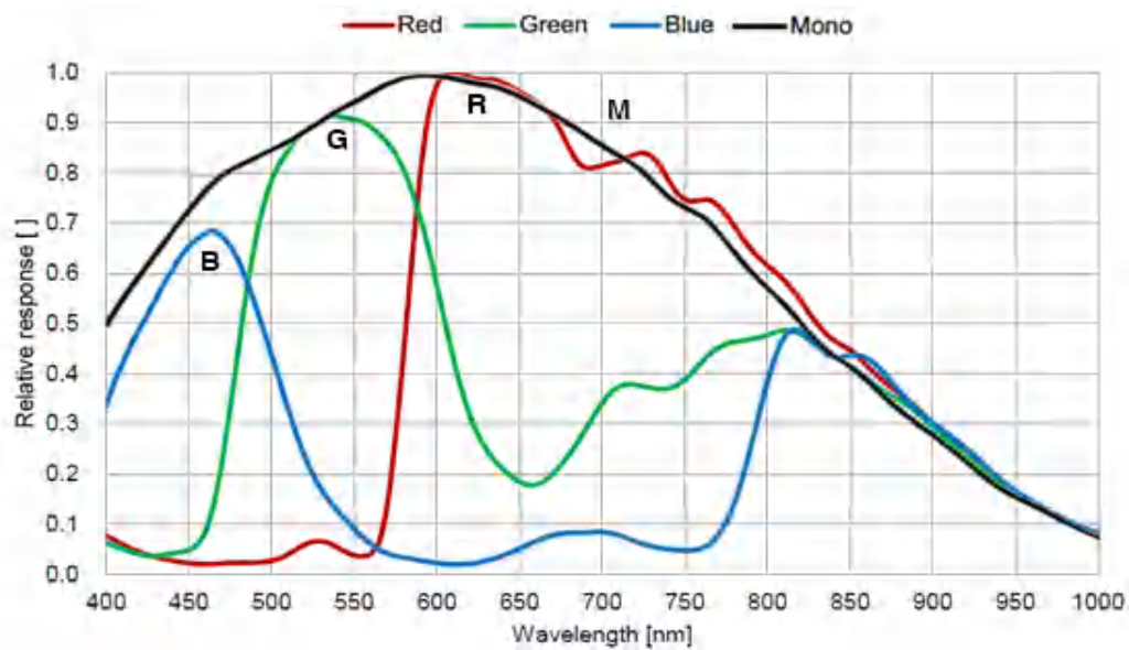
图 4-25 MER2-041-608U3M/C(-L)-HS SENSOR 响应曲线
