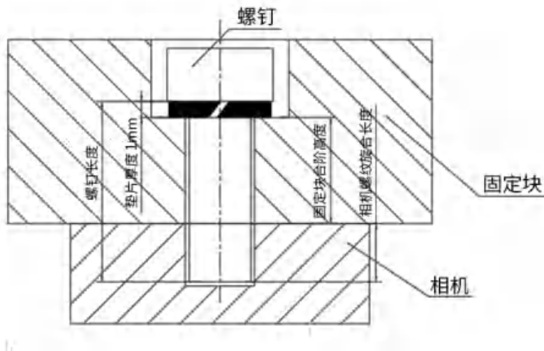
图 5-13 螺钉规格、固定块台阶厚度、弹垫厚度关系图
