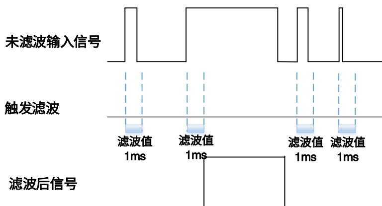
图 8-1 输入信号滤波示意图
