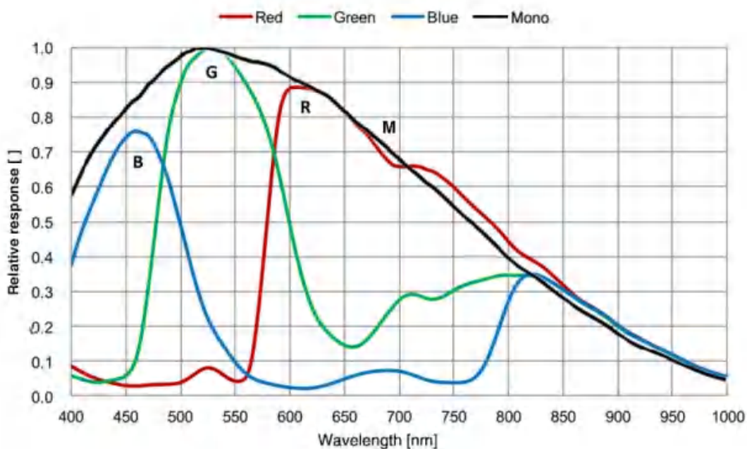
图 4-8 MER2-231-41U3M/C(-L) SENSOR 响应曲线
