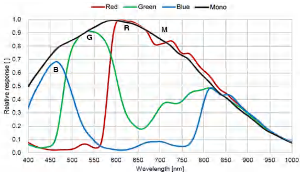
图 4-30 MER2-041-608U3M/C(-L)-HS-6P SENSOR 响应曲线
