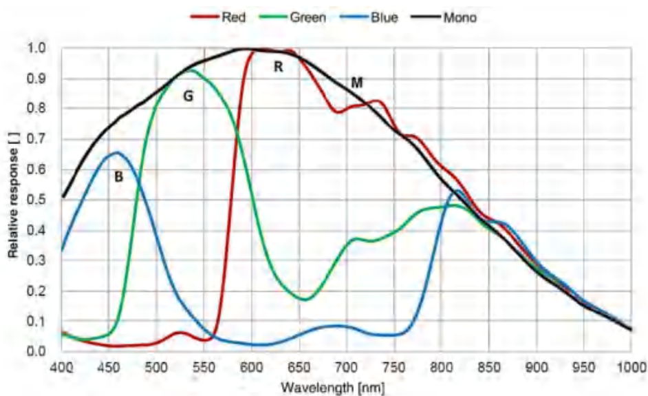
图 4-20 MER2-510-36U3M/C(-L) SENSOR 响应曲线
