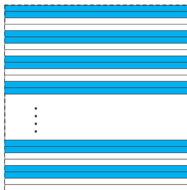
图 8-53 彩色相机垂直像素抽样原理
