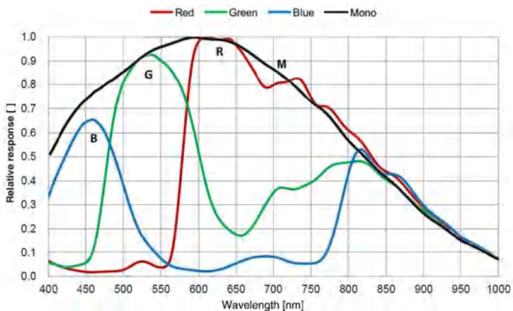
图 4-12 MER2-302-56U3M/C(-L) SENSOR 响应曲线
