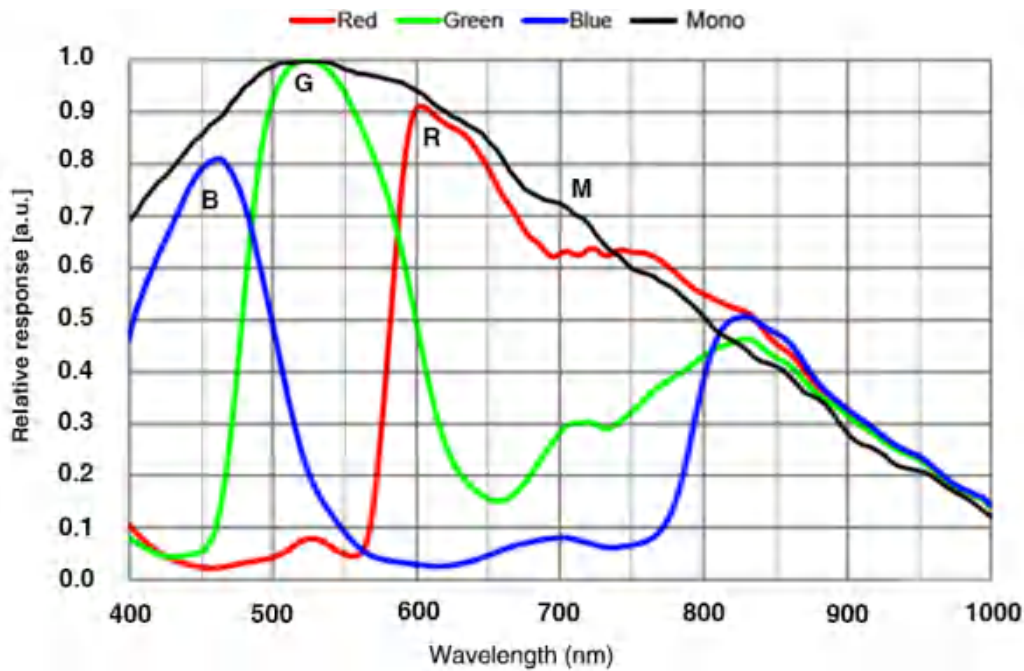
图 4-58 ME2L-505-36U3M/C(-L) SENSOR 响应曲线
