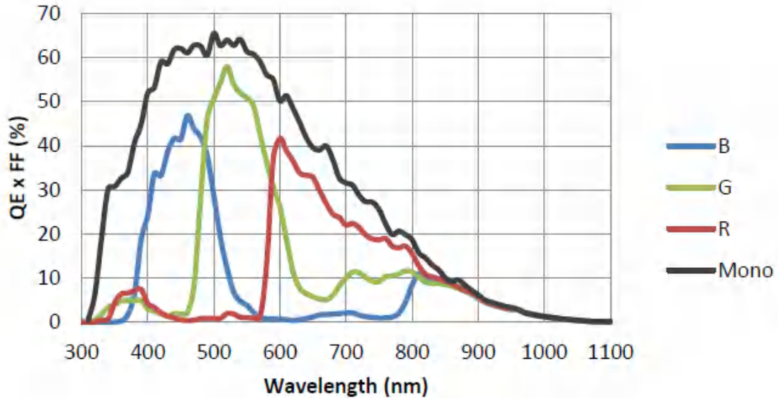
图 4-43 ME2P-560-36U3M/C SENSOR 响应曲线
