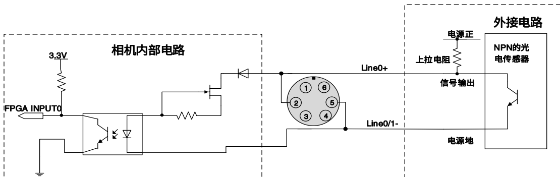
图 7-5 NPN 型光电传感器连接到光耦隔离输入电路 (MER2-6P/ME2S)
