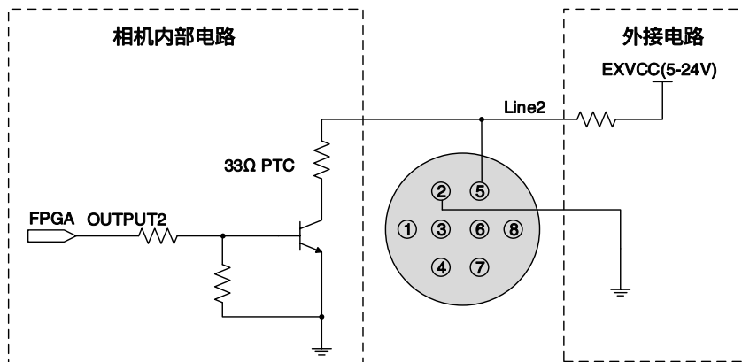
图 7-25 Line2 配置为输出引脚时相机内部等效电路 (MER2/ME2P/ME2L)
