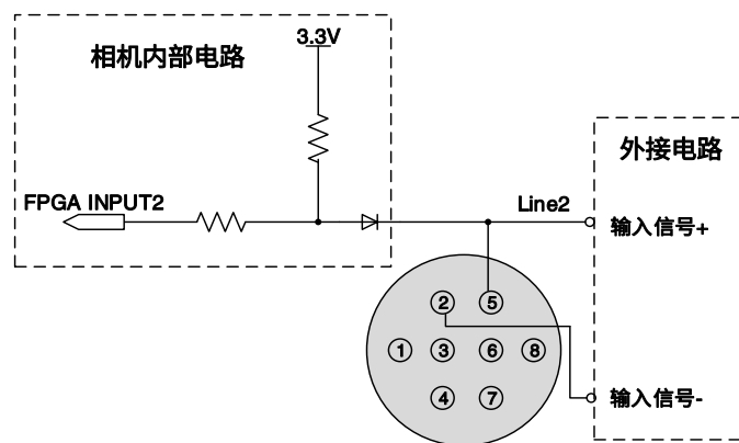
图 7-14 Line2 配置为输入引脚时相机内部等效电路 (MER2/ME2P)
