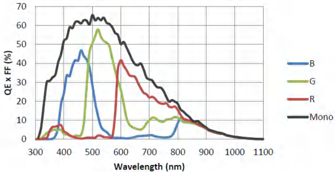
图 4-45 ME2P-900-43U3M/C SENSOR 响应曲线
