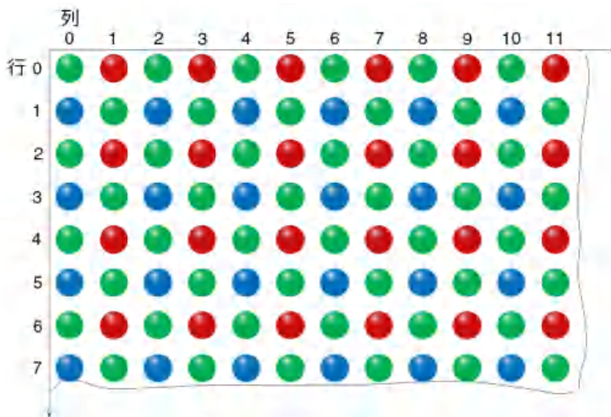
图 8-40 BayerGR8 的像素排列示意图
