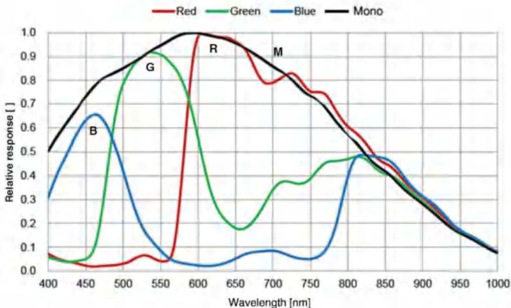
图 4-6 MER2-160-227U3M/C(-L) SENSOR 响应曲线
