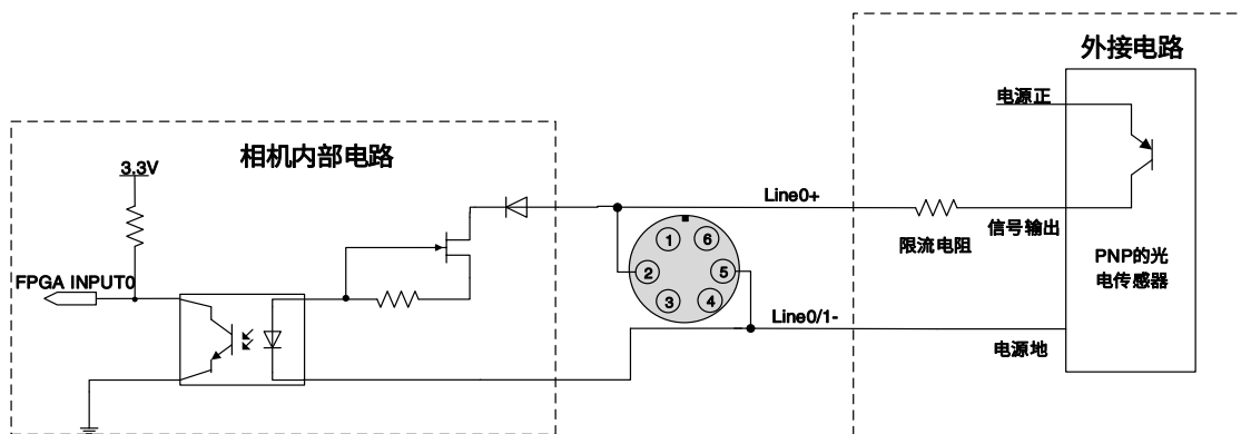
图 7-6 PNP 型光电传感器连接到光耦隔离输入电路 (MER2-6P/ME2S)
