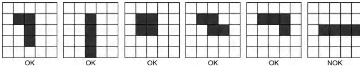
图 4-51 ME2P-2622-15U3M 连续坏点分布情况示意图
