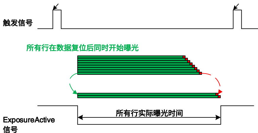
图 8-10 全局复位释放曝光模式 ExposureActive 信号示意图
