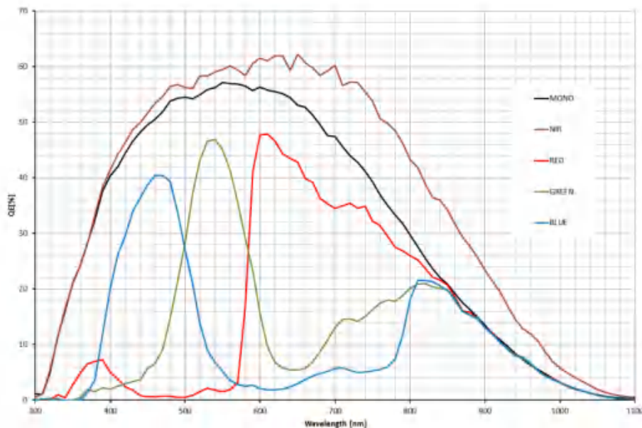
图 4-42 ME2P-530-72U3M NIR \ ME2P-530-72U3C SENSOR 响应曲线
