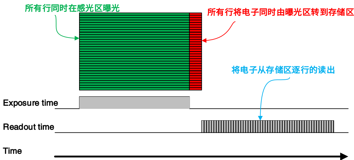
图 8-32 全局曝光模式
