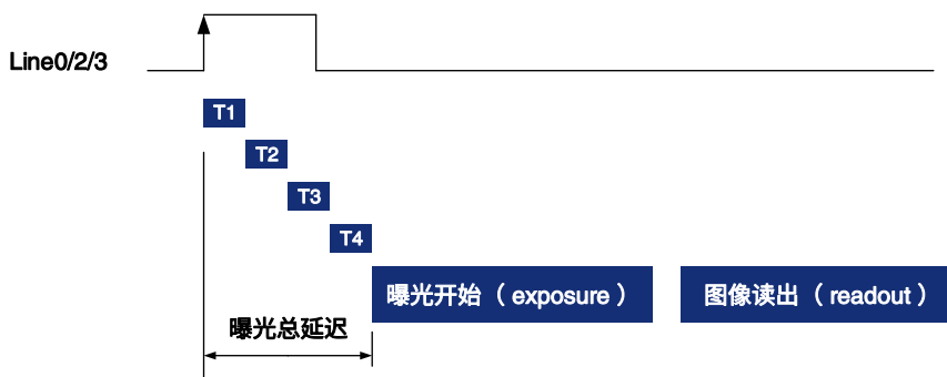
图 8-36 曝光延迟
