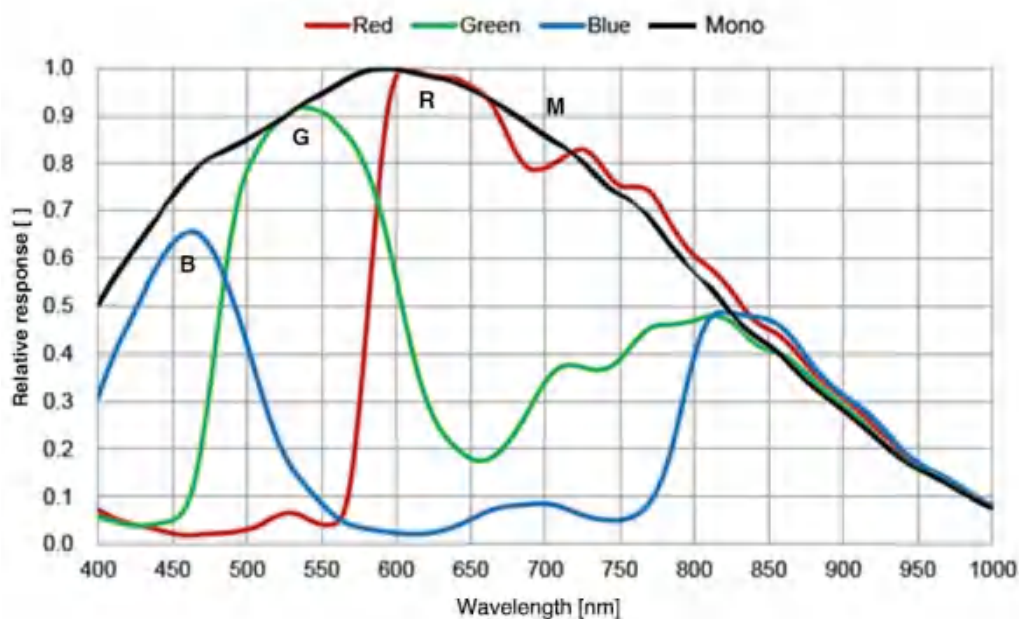
图 4-26 MER2-160-249U3M/C(-L)-HS SENSOR 响应曲线
