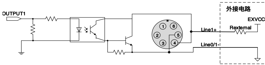
图 7-9 光耦隔离输出电路 (MER2-6P/ME2S)
