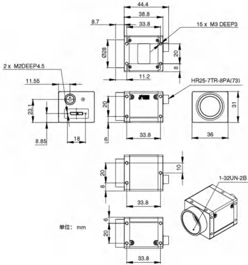
图 5-9 ME2P-U3 机械尺寸图
