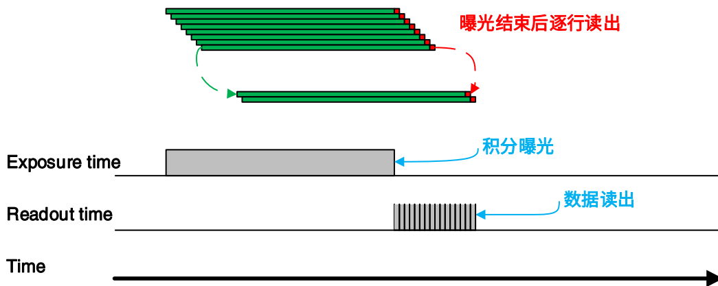
图 8-33 逐行曝光模式
