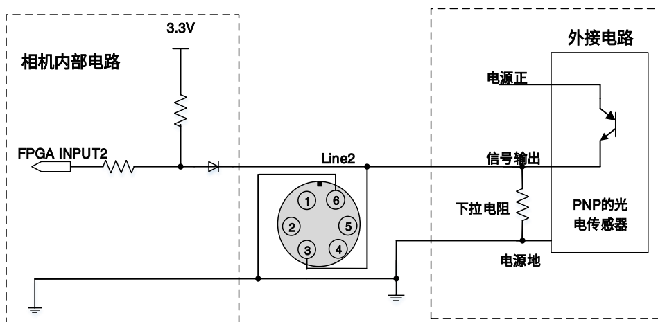
图 7-22 PNP 型光电传感器连接到 Line2 输入电路 (MER2-6P/ME2S)
