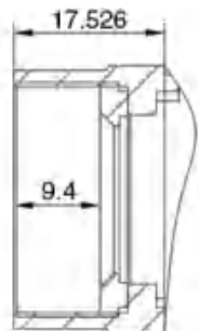
图 5-11 ME2L C 口光学接口
