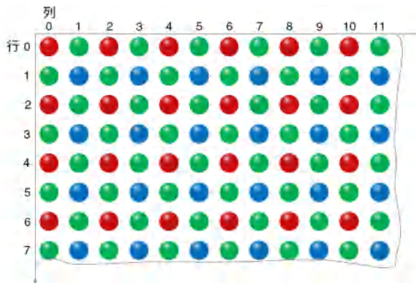
图 8-39 BayerRG8 的像素排列示意图
