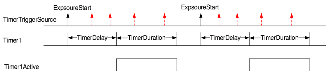
图 8-67 Timer1Active 与曝光开始信号的关系
