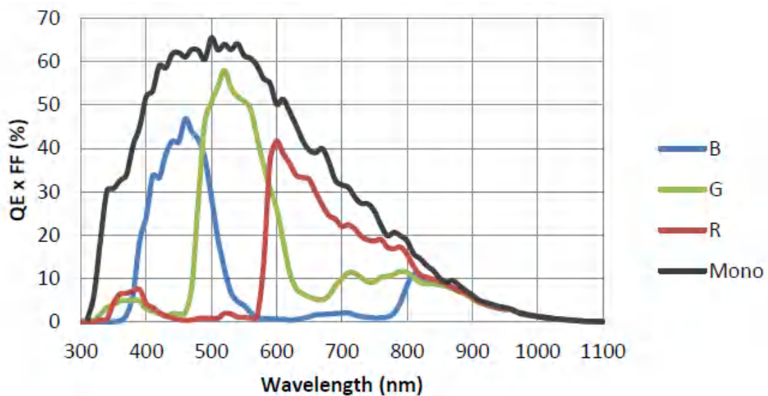
图 4-32 ME2S-560-70U3M/C SENSOR 响应曲线
