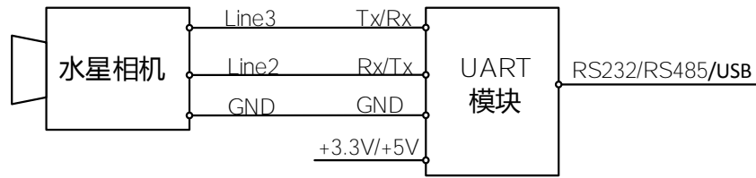
图 8-101 相机和外部串口设备的接线图
