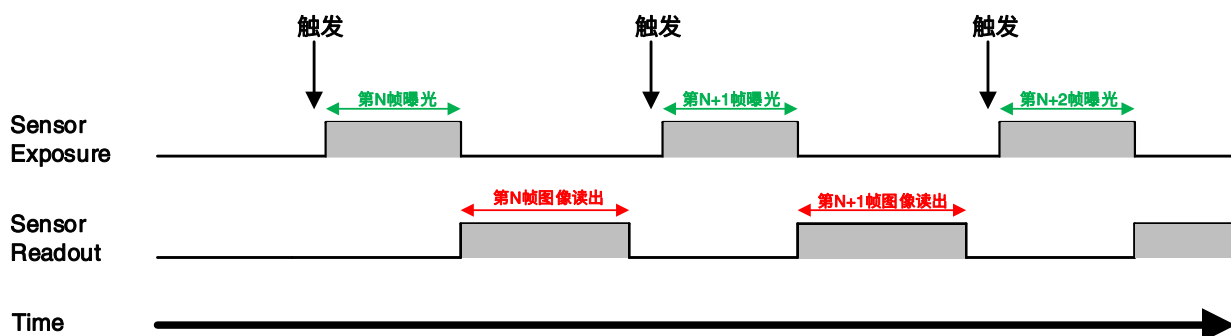
图 8-25 非交叠曝光模式下触发采集曝光时序图
