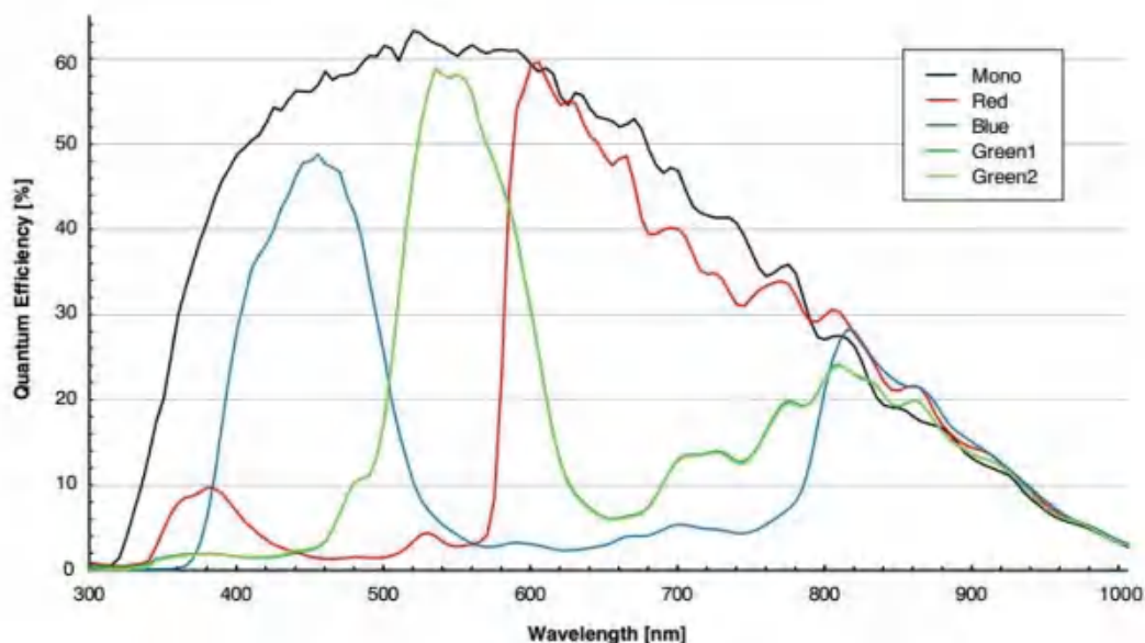
图 4-33 ME2S-1260-28U3M/C SENSOR 响应曲线
