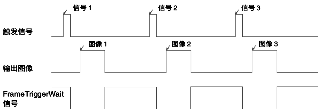
图 8-11 FrameTriggerWait 信号示意图
