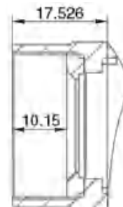
图 5-12 ME2S C 口光学接口
