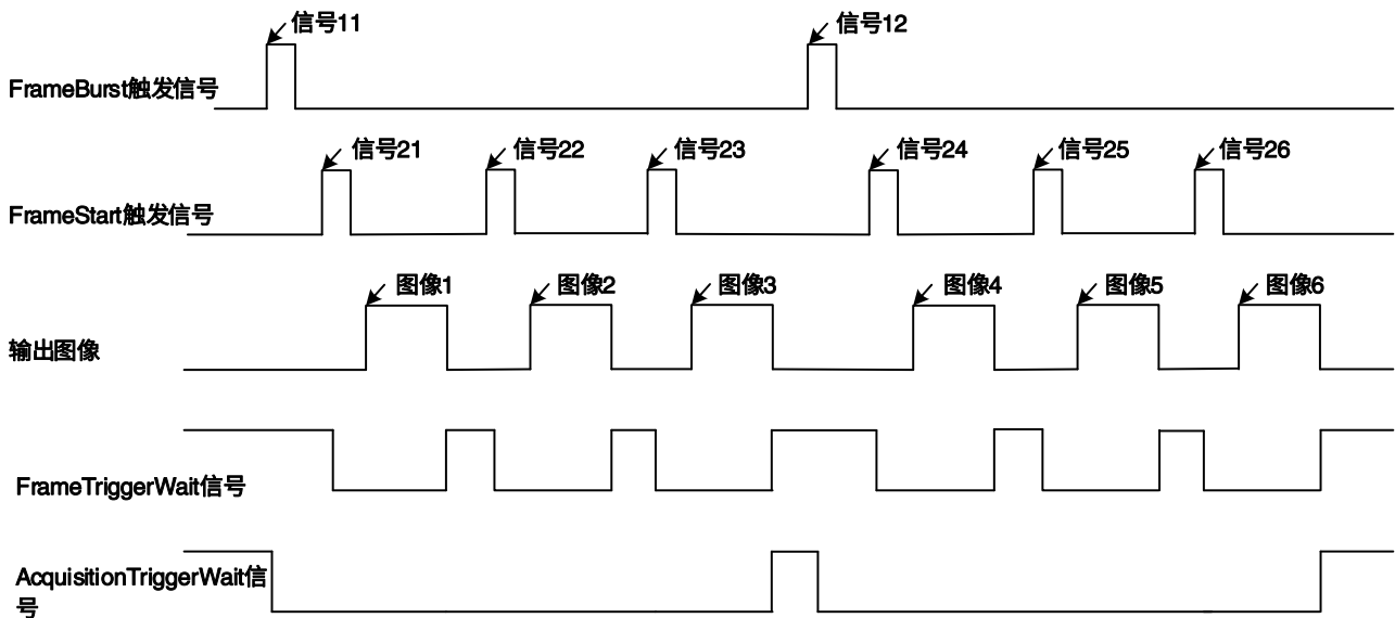
图 8-13 FrameBurstStart、FrameStart 同时使能时 TriggerWait 信号示意图
