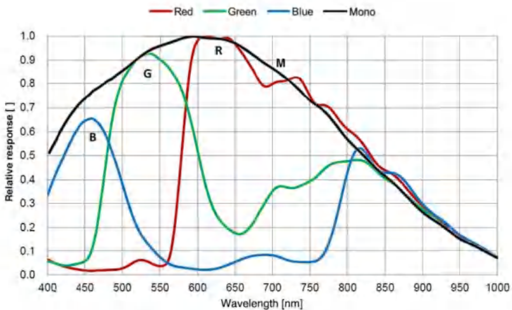
图 4-28 MER2-502-79U3M/C(-L)-HS SENSOR 响应曲线
