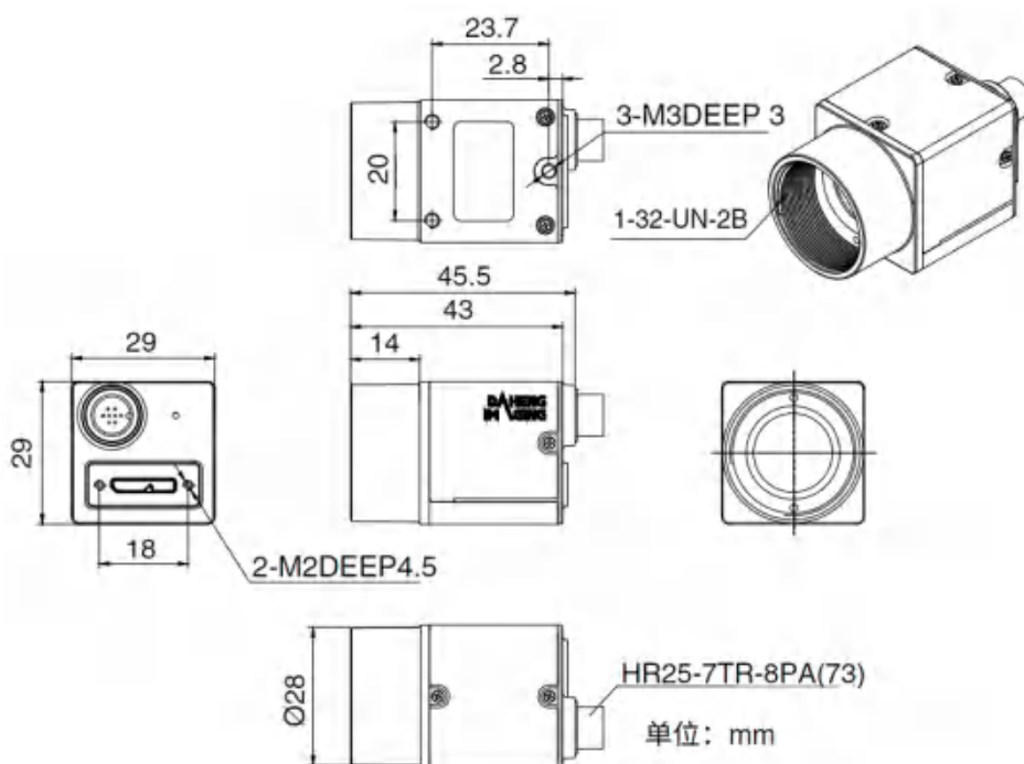
图 5-1 MER2-U3 机械尺寸图
