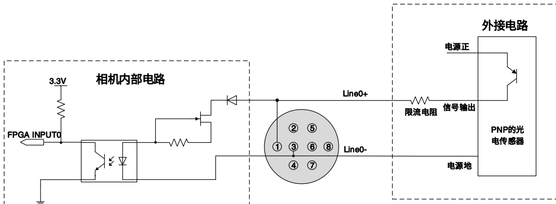
图 7-4 PNP 型光电传感器连接到光耦隔离输入电路 (MER2/ME2P/ME2L)
