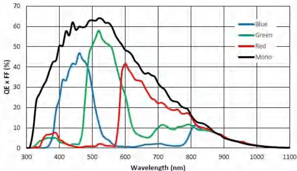
图 4-49 ME2P-1840-21U3M/C SENSOR 响应曲线
