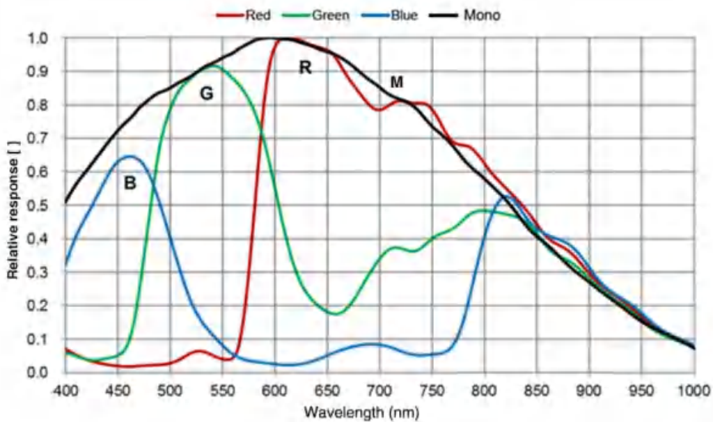
图 4-46 ME2P-1230-23U3M/C SENSOR 响应曲线
