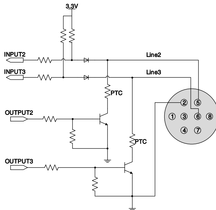
图 7-11 Line2/3 (双向) 电路 (MER2/ME2P)
