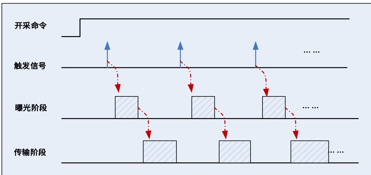
图 8-16 触发采集时序图
