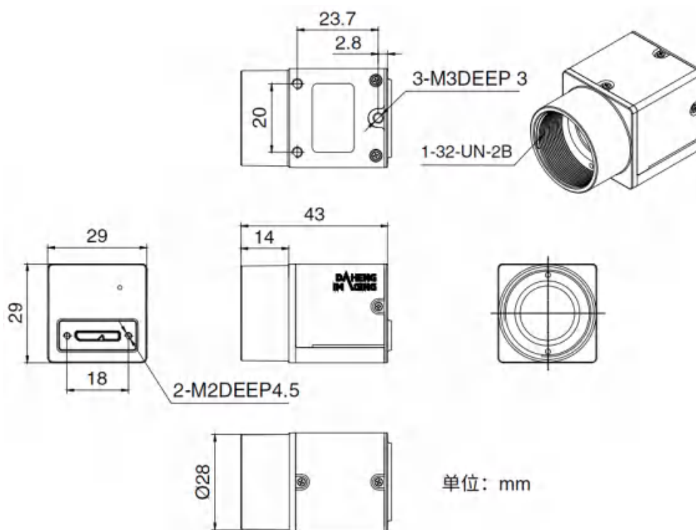
图 5-6 MER2-U3-L-6P 机械尺寸图
