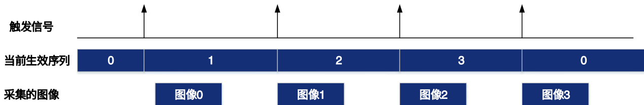
图 8-103 当前生效序列与触发信号和采集图像的关系
