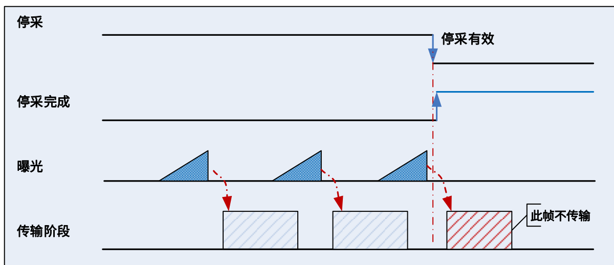
图 8-18 传输等待时停采时序图
