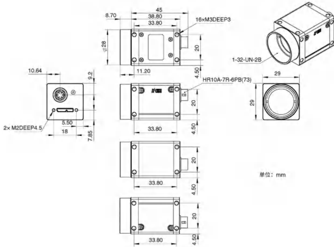
图 5-7 ME2S-U3 机械尺寸图
