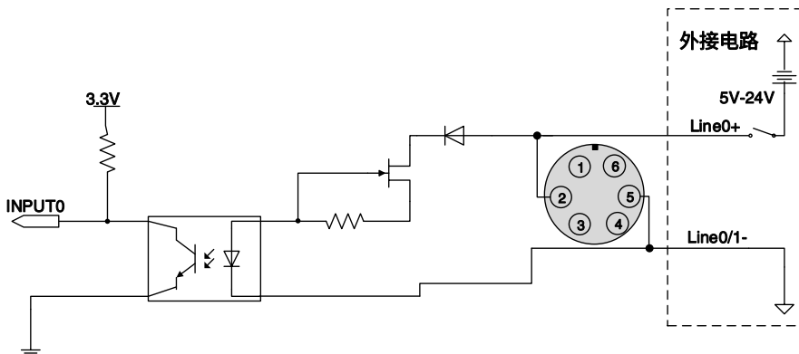
图 7-2 光耦隔离输入电路 (MER2-6P/ME2S)
