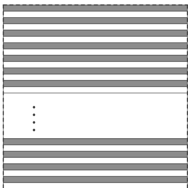
图 8-52 黑白相机垂直像素抽样原理
