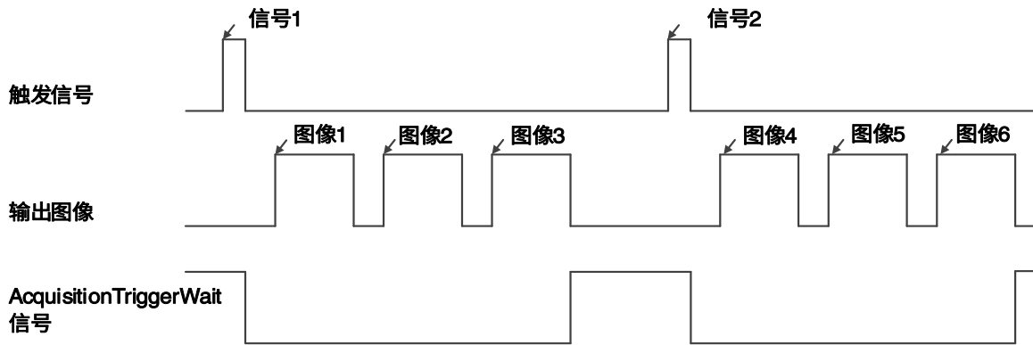
图 8-12 AcquisitionTriggerWait 信号示意图
