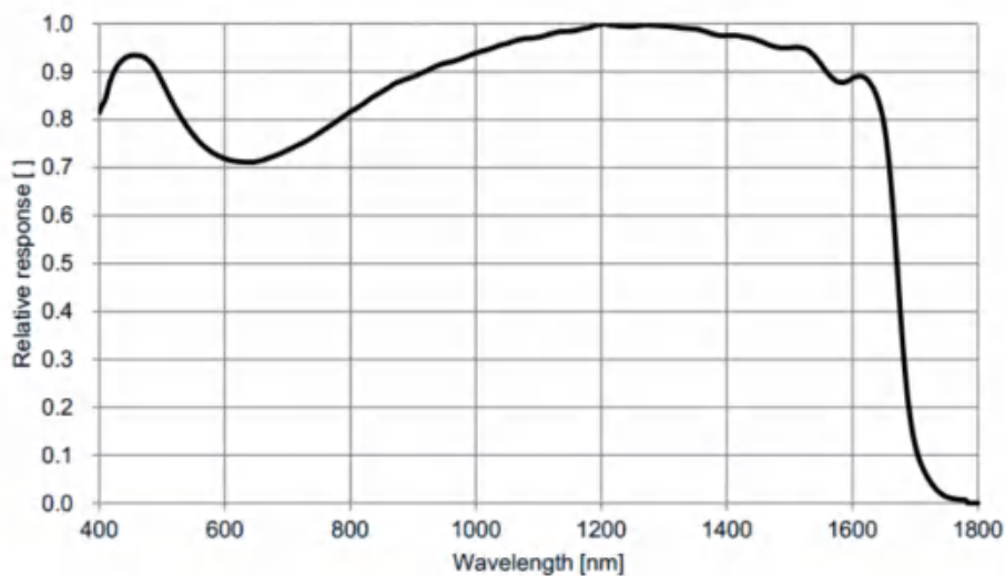
图 4-40 ME2S-138-232U3M-SWIR SENSOR 响应曲线
