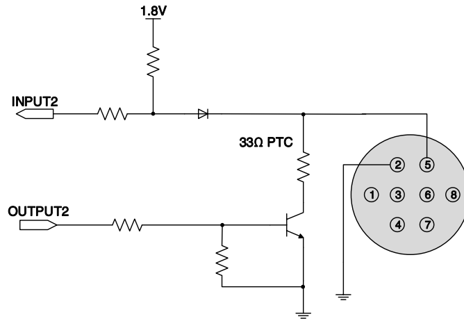
图 7-12 Line2 (双向) 电路 (ME2L)
