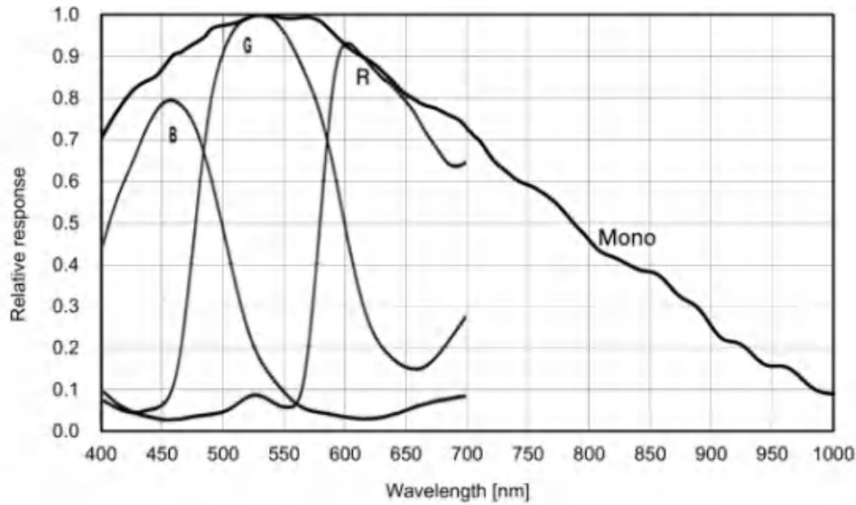
图 4-23 MER2-2000-19U3M/C(-L/-W90/-W90-S90) SENSOR 响应曲线
