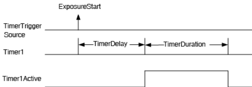
图 8-66 Timer1Active 示意图
