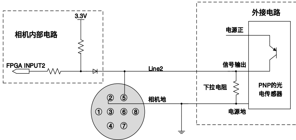
图 7-18 PNP 型光电传感器连接到 Line2 输入电路 (MER2/ME2P)
