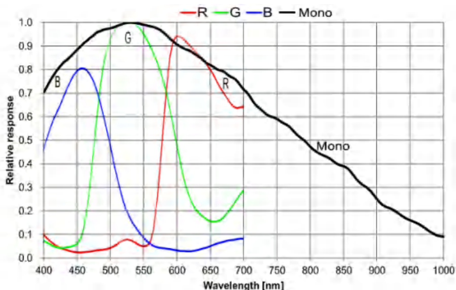
图 4-21 MER2-630-60U3M/C(-L/-W90/-W90-S90) SENSOR 响应曲线
