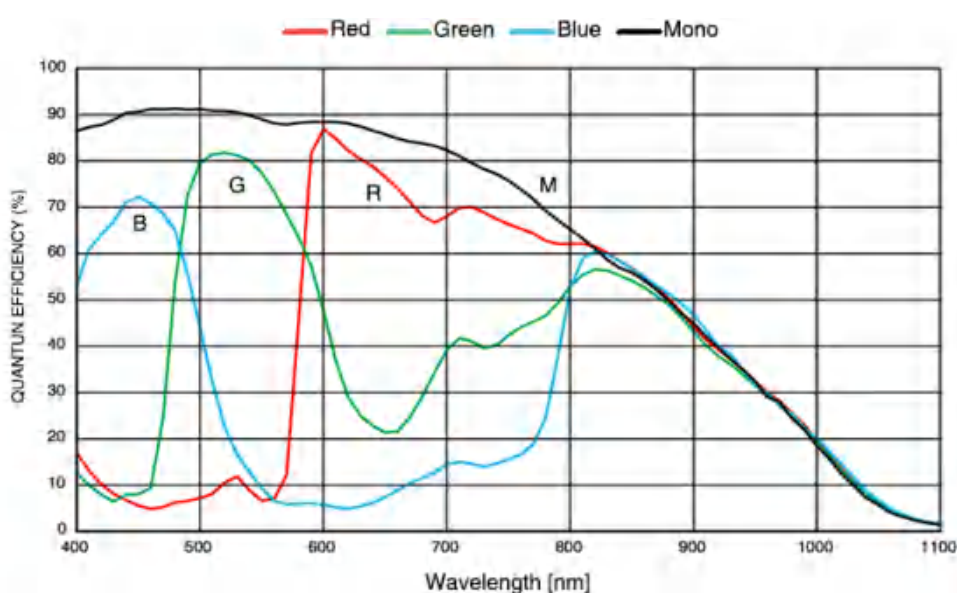
图 4-24 MER2-2002-20U3M/C(-L) SENSOR 响应曲线
