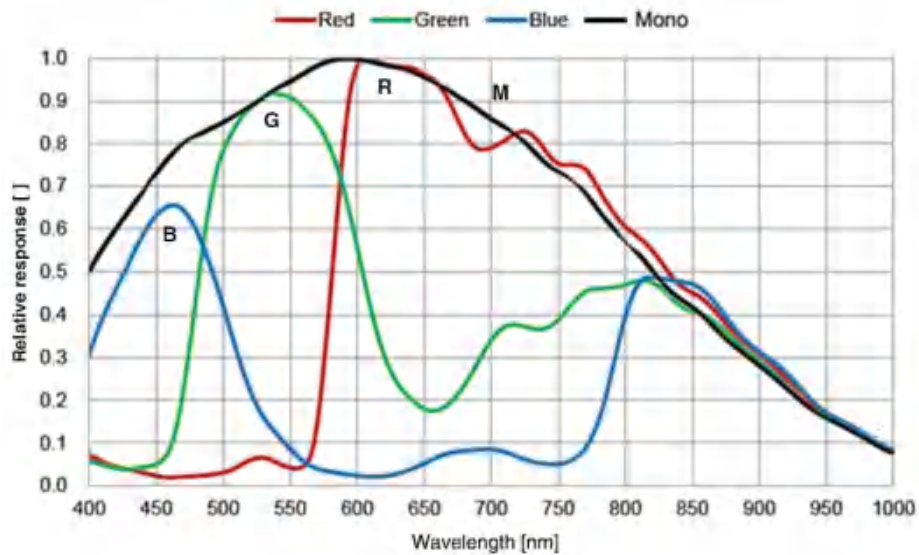
图 4-31 MER2-160-249U3M/C(-L)-HS-6P SENSOR 响应曲线
