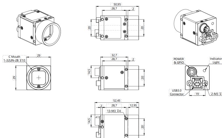
SUA-T1V-C
