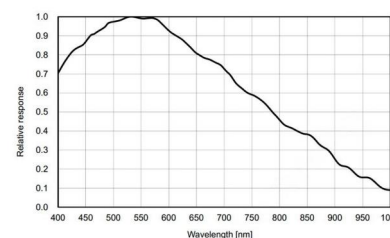
MV-SUA2000M
