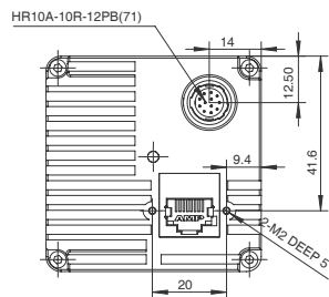
A向视图
