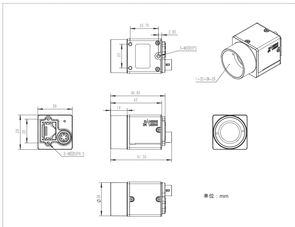
ME2C-2000-6GM/C
