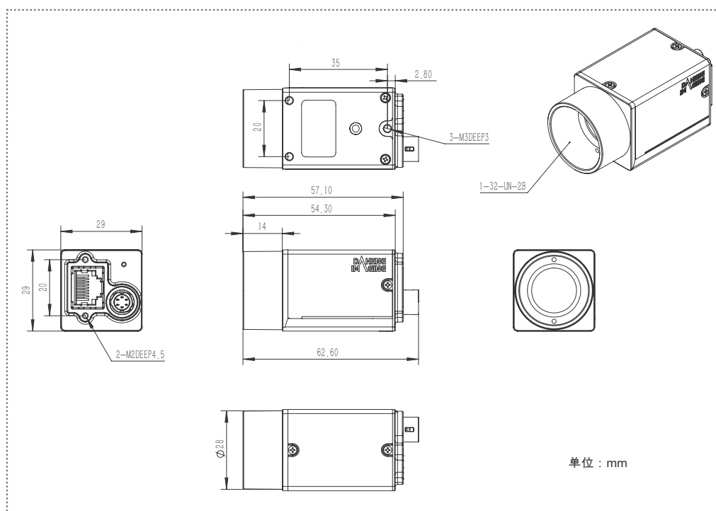
ME2C-2000-6GM/C-P
