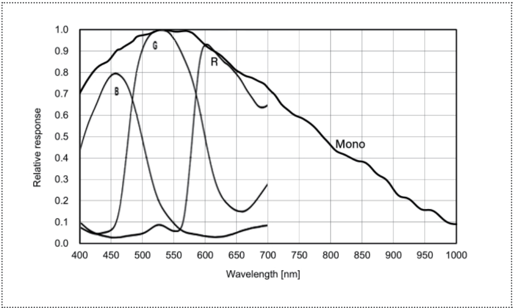
ME2C-2000-6GM/C ME2C-2000-6GM/C-P
