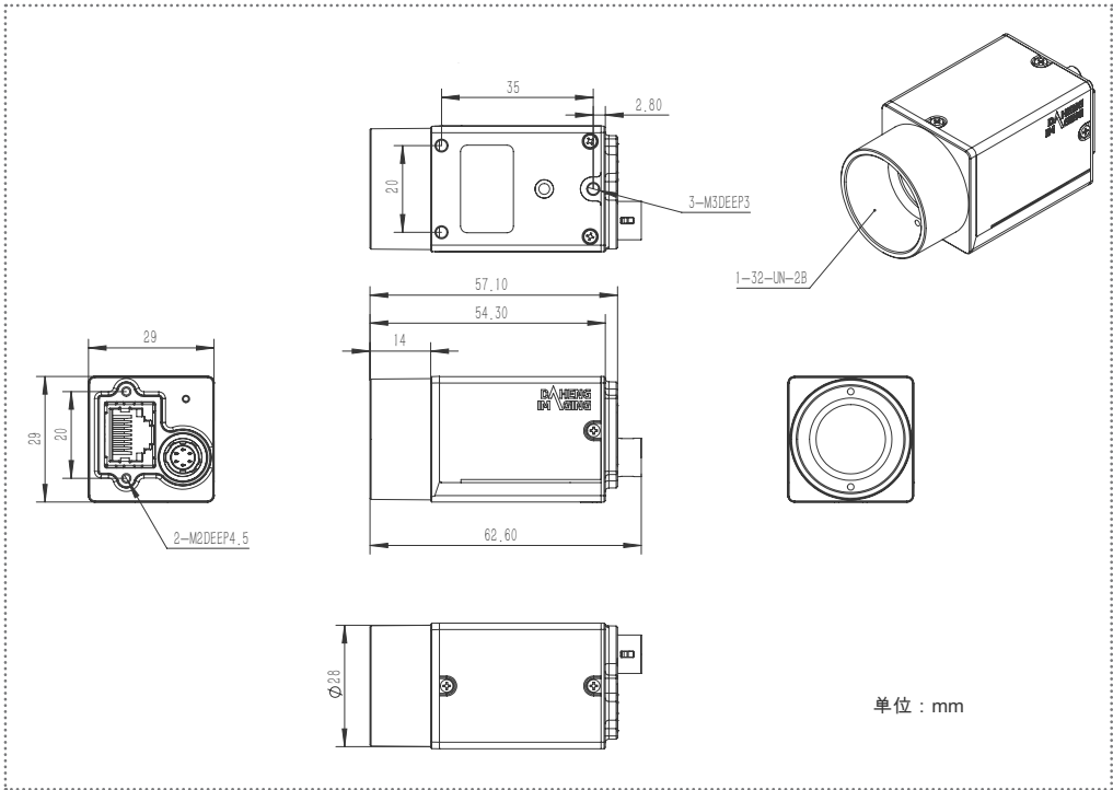
ME2C-202-60GM/C-P
