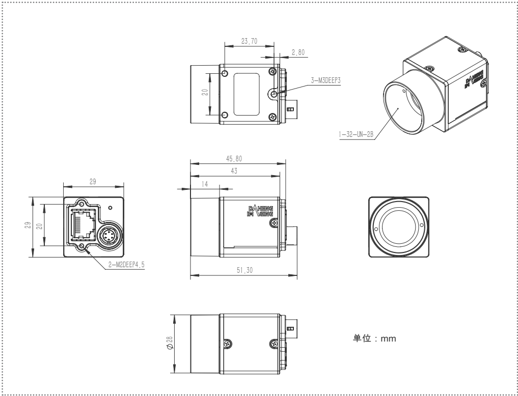
ME2C-202-60GM/C
