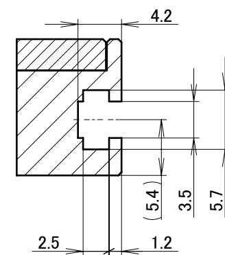
M3ナットスロット詳細図 _Nut slot Detail drawing
