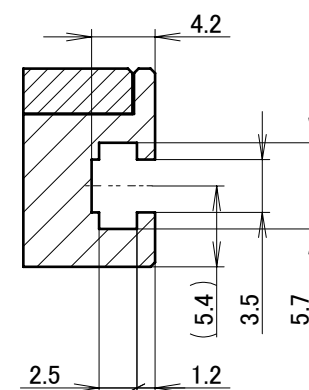
M3ナットスロット詳細図 _Nut slot Detail drawing
