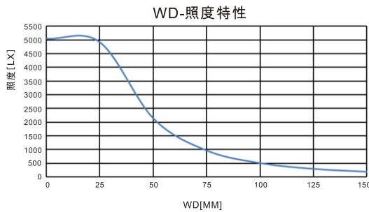
照度特性图
