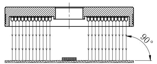
照明示意图
