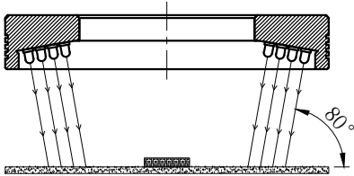
照明示意图
