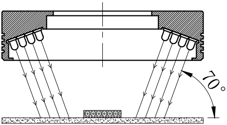
照明示意图
