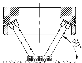
照明示意图
