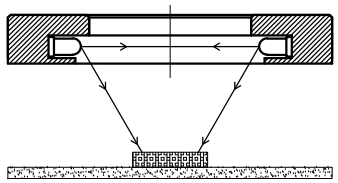
照明示意图
