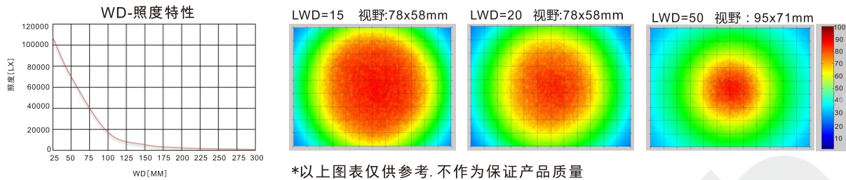
照度特性图
