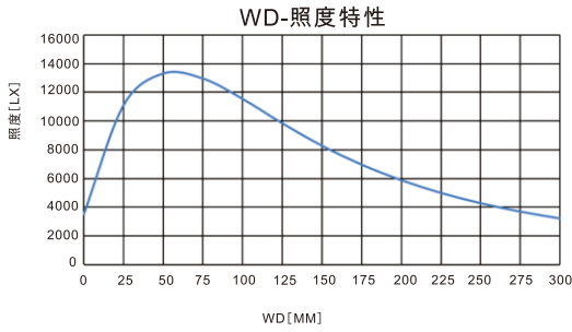
照度特性图
