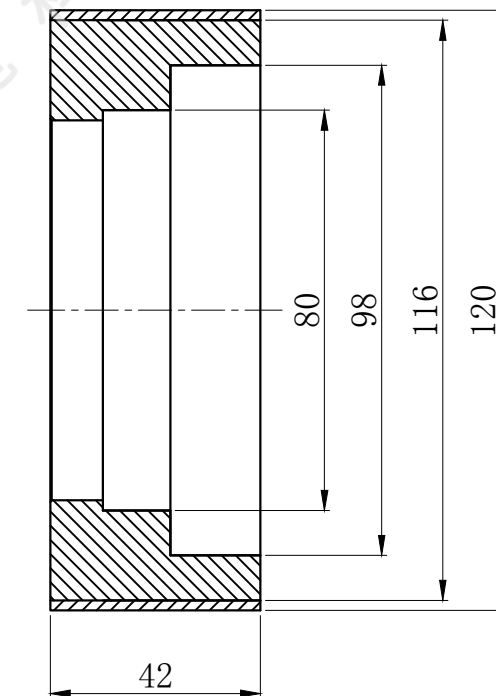
SECTION A-A
