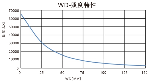
照度特性图
