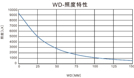
照度特性图
