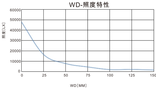
照度特性图
