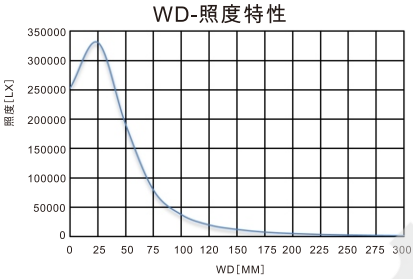
照度特性图
