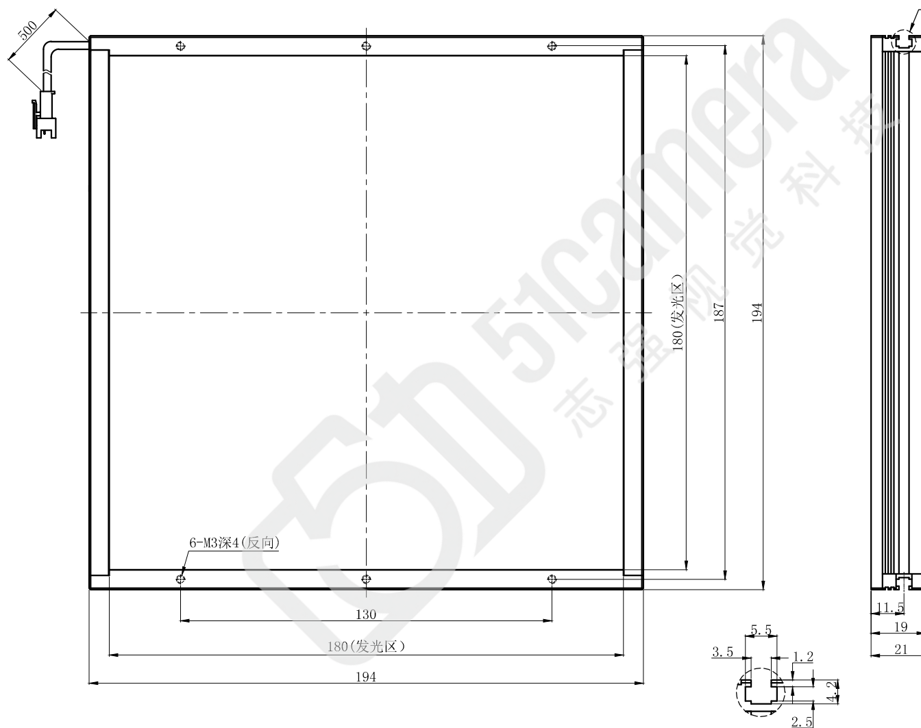
视图A, 比例2:1
