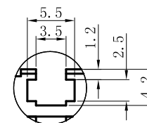
视图A, 比例2:1
