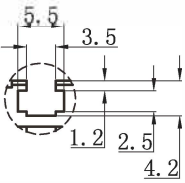
视图A，比例2:1
