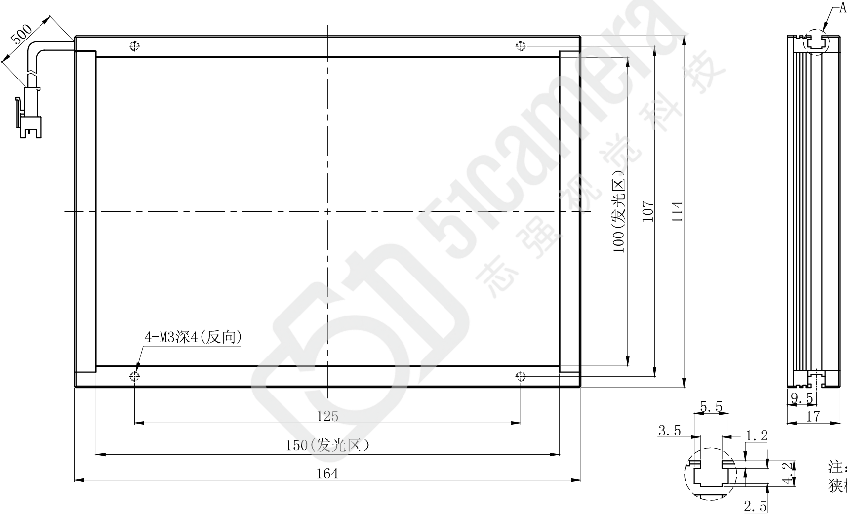
视图A，比例2:1
