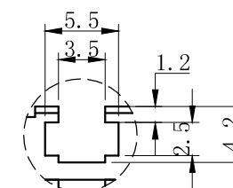
视图A, 比例2:1
