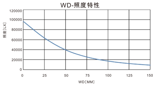
照度特性图
