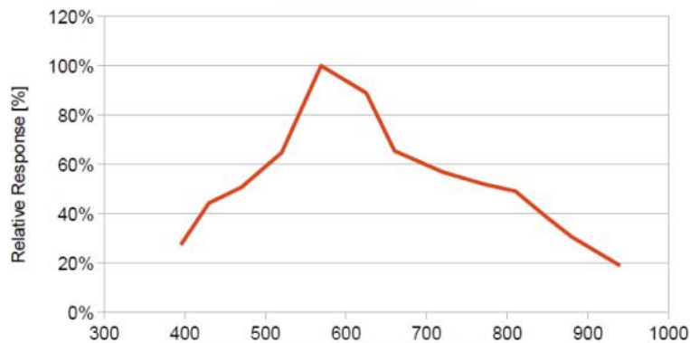
相机光谱响应曲线
