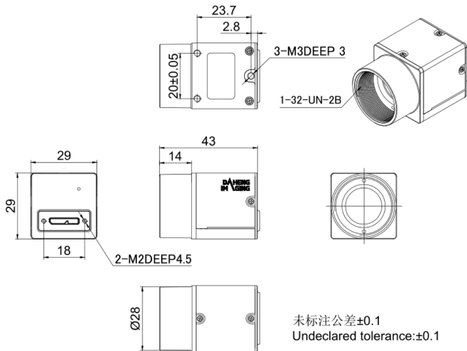
MER2-U3-L 机械尺寸图
