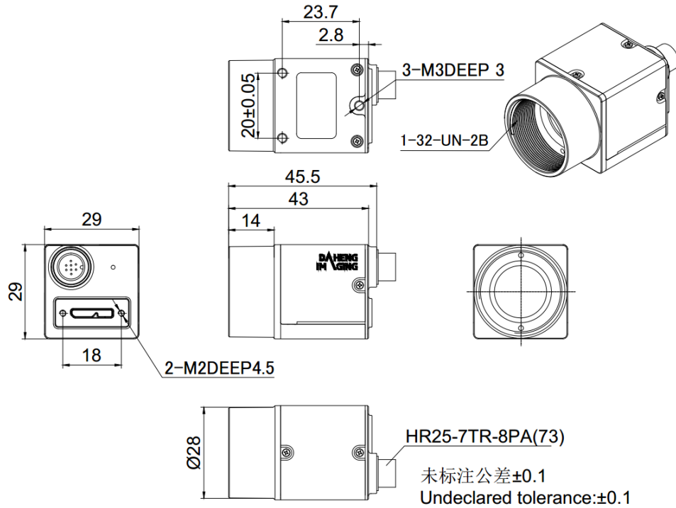
MER2-U3 机械尺寸图
