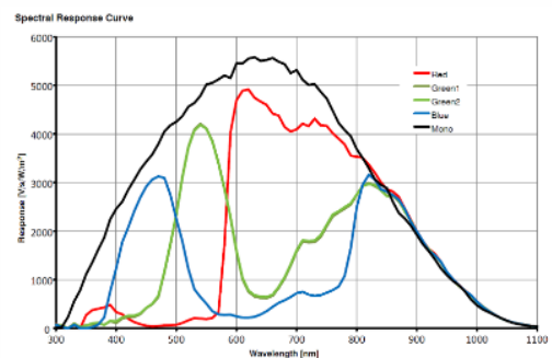
MV-CA003-21UM/UC 量子效率
