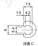
详图 C
